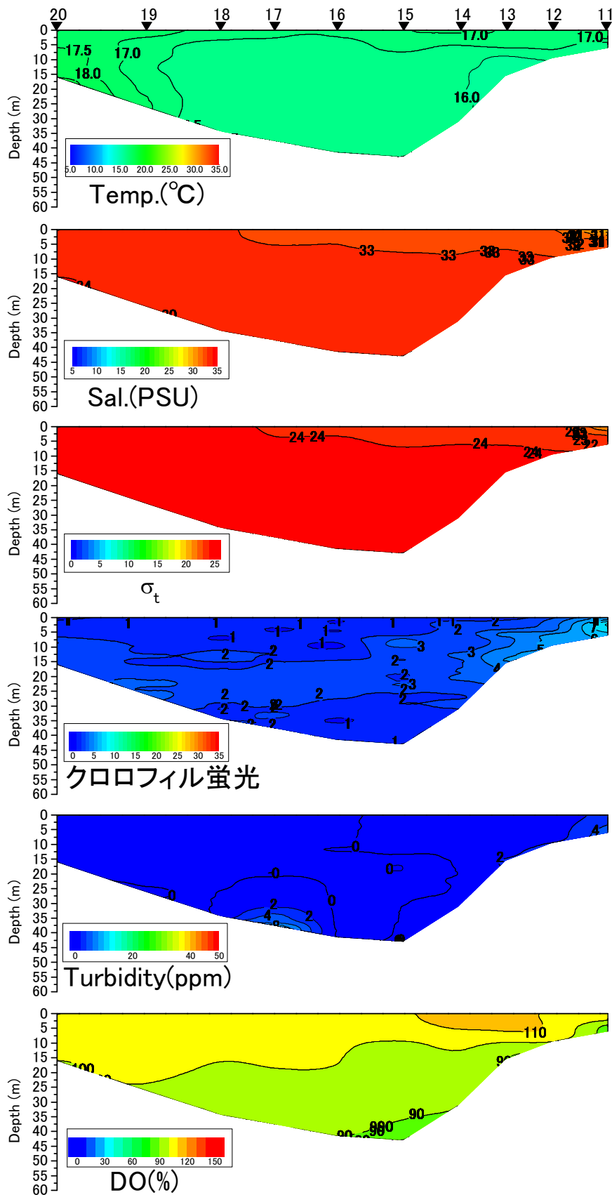
八代海中央ラインの水温(°C)、塩分、密度( \sigma_t )、クロロフィル蛍光強度、濁度、溶存酸素飽和度(DO%)の鉛直面図(国土交通省の調査による) (2014年4月25日)
