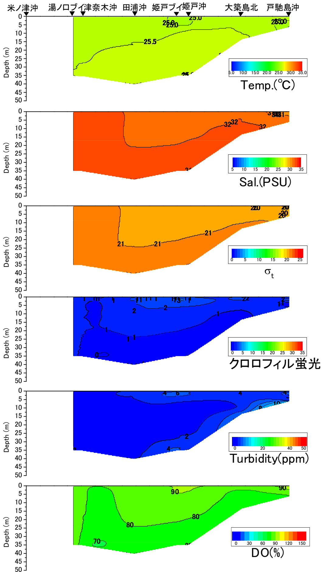
戸馳島沖から米ノ津沖の水温(°C)、塩分、密度( \sigma_t )、クロロフィル蛍光強度、濁度、溶存酸素飽和度(DO%)の鉛直面図(東町漁業協同組合の調査による) (2013年9月27日)
