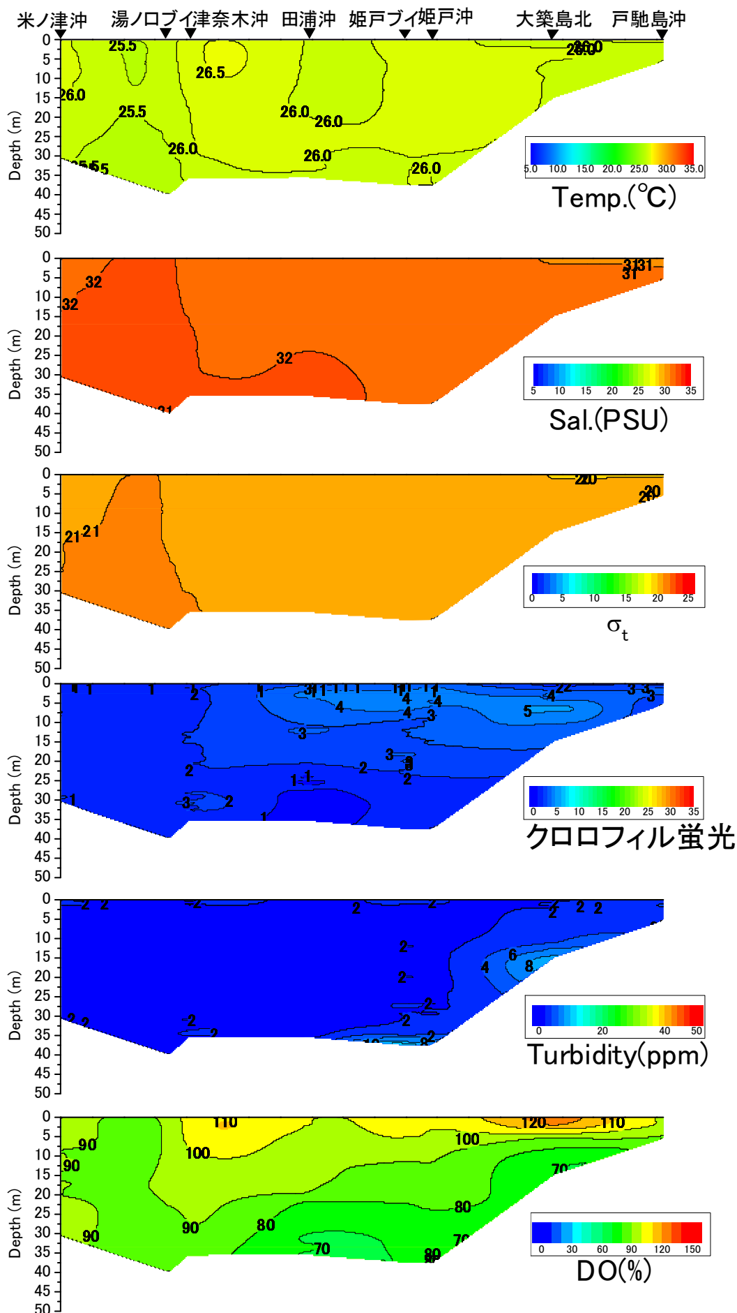
戸馳島沖から米ノ津沖の水温(°C)、塩分、密度( \sigma_t )、クロロフィル蛍光強度、濁度、溶存酸素飽和度(DO%)の鉛直面図(東町漁業協同組合の調査による) (2013年9月19日)
