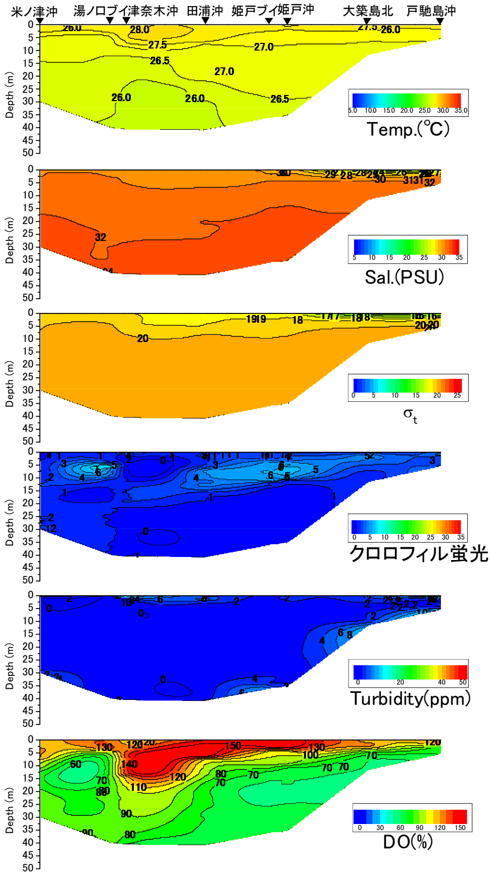
戸馳島沖から米ノ津沖の水温(°C)、塩分、密度( \sigma_t )、クロロフィル蛍光強度、濁度、溶存酸素飽和度(DO%)の鉛直面図(東町漁業協同組合の調査による) (2013年9月12日)
