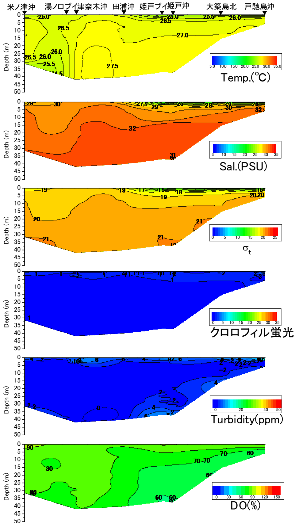
戸馳島沖から米ノ津沖の水温(°C)、塩分、密度( \sigma_t )、クロロフィル蛍光強度、濁度、溶存酸素飽和度(DO%)の鉛直面図(東町漁業協同組合の調査による) (2013年9月5日)
