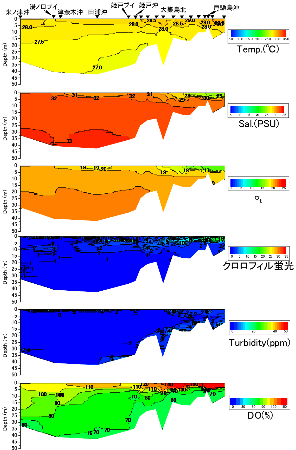
戸馳島沖から米ノ津沖の水温(°C)、塩分、密度( \sigma_t )、クロロフィル蛍光強度、濁度、溶存酸素飽和度(DO%)の鉛直面図(東町漁業協同組合、熊本県水産研究センター、西海区水産研究所の調査による)(2013年8月29日)
