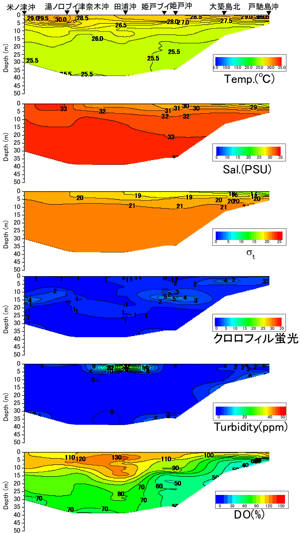
戸馳島沖から米ノ津沖の水温(°C)、塩分、密度( \sigma_t )、クロロフィル蛍光強度、濁度、溶存酸素飽和度(DO%)の鉛直面図(東町漁業協同組合の調査による) (2013年8月16日)
