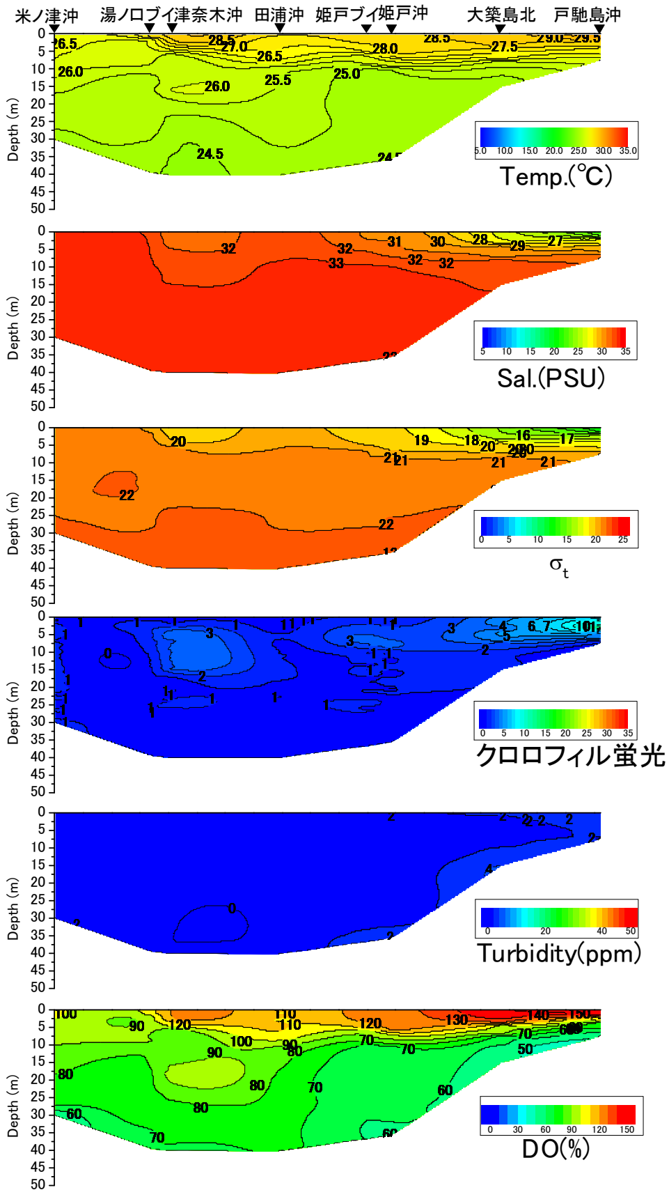
戸馳島沖から米ノ津沖の水温(°C)、塩分、密度( \sigma_t )、クロロフィル蛍光強度、濁度、溶存酸素飽和度(DO%)の鉛直面図(東町漁業協同組合の調査による) (2013年8月8日)
