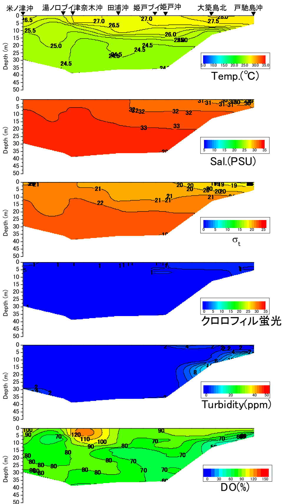
戸馳島沖から米ノ津沖の水温(°C)、塩分、密度( \sigma_t )、クロロフィル蛍光強度、濁度、溶存酸素飽和度(DO%)の鉛直面図(東町漁業協同組合の調査による) (2013年7月31日)
