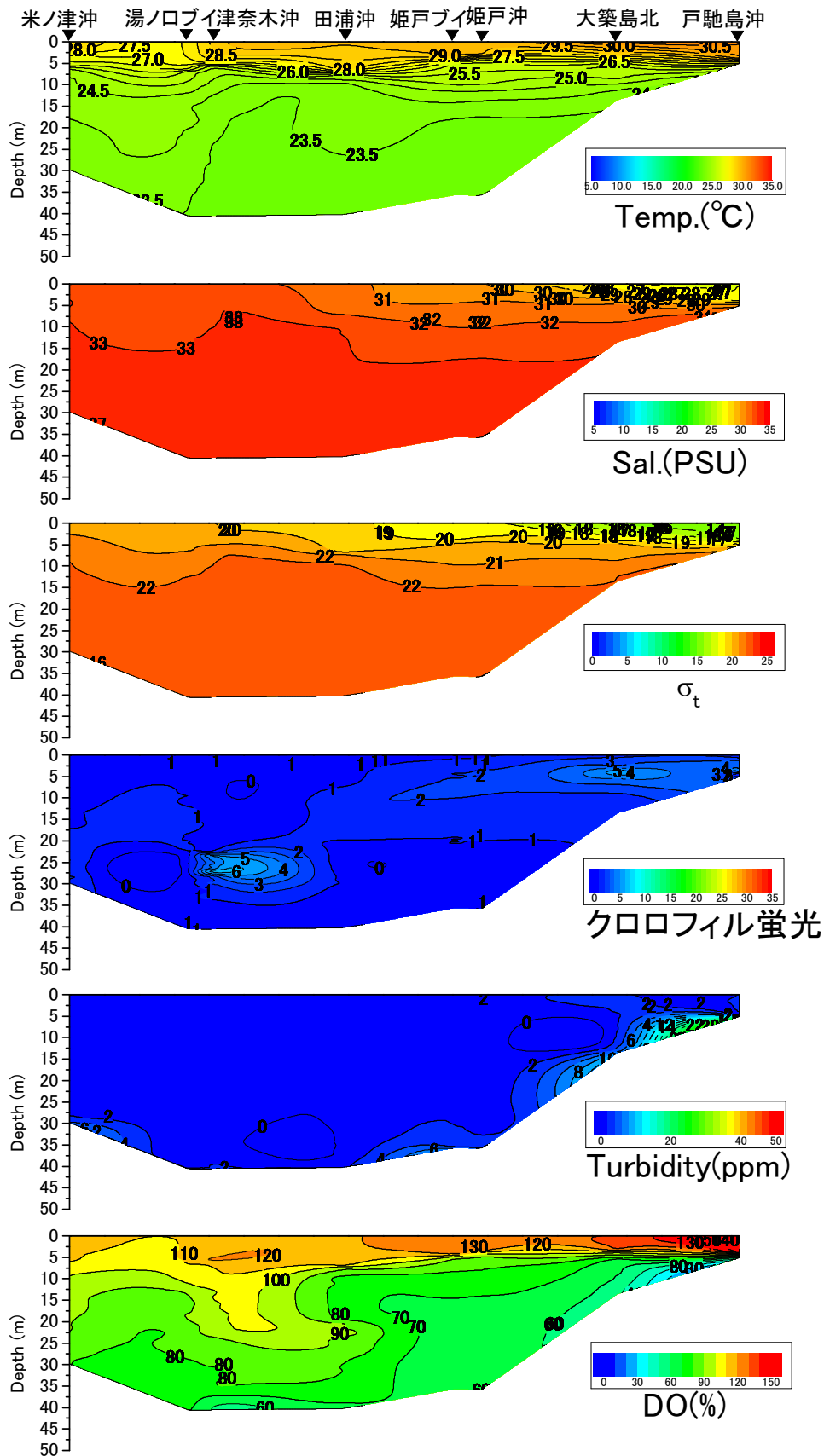
戸馳島沖から米ノ津沖の水温(°C)、塩分、密度( \sigma_t )、クロロフィル蛍光強度、濁度、溶存酸素飽和度(DO%)の鉛直面図(東町漁業協同組合の調査による) (2013年7月19日)
