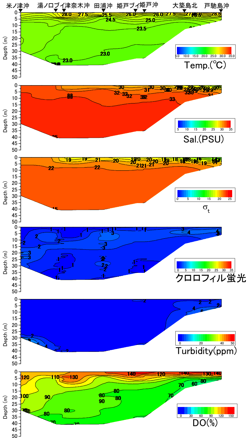
戸馳島沖から米ノ津沖の水温(°C)、塩分、密度( \sigma_t )、クロロフィル蛍光強度、濁度、溶存酸素飽和度(DO%)の鉛直面図(東町漁業協同組合の調査による) (2013年7月12日)
