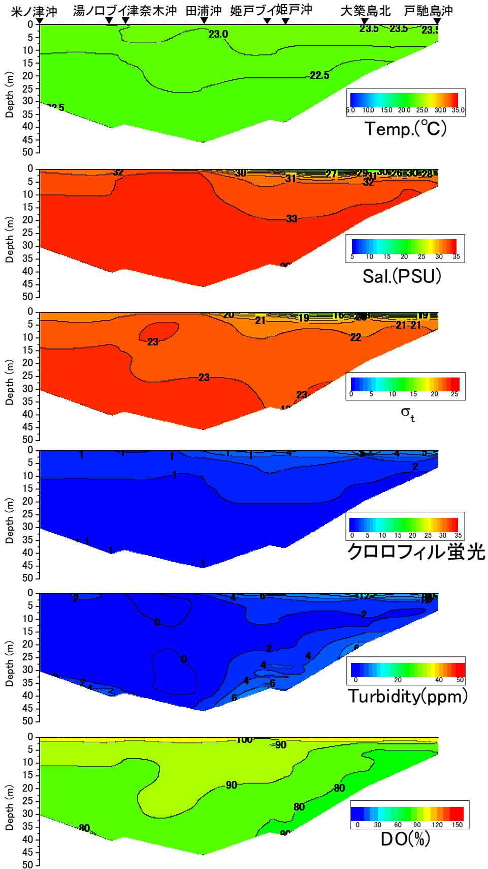
戸馳島沖から米ノ津沖の水温(°C)、塩分、密度( \sigma_t )、クロロフィル蛍光強度、濁度、溶存酸素飽和度(DO%)の鉛直面図(東町漁業協同組合の調査による) (2013年6月27日)
