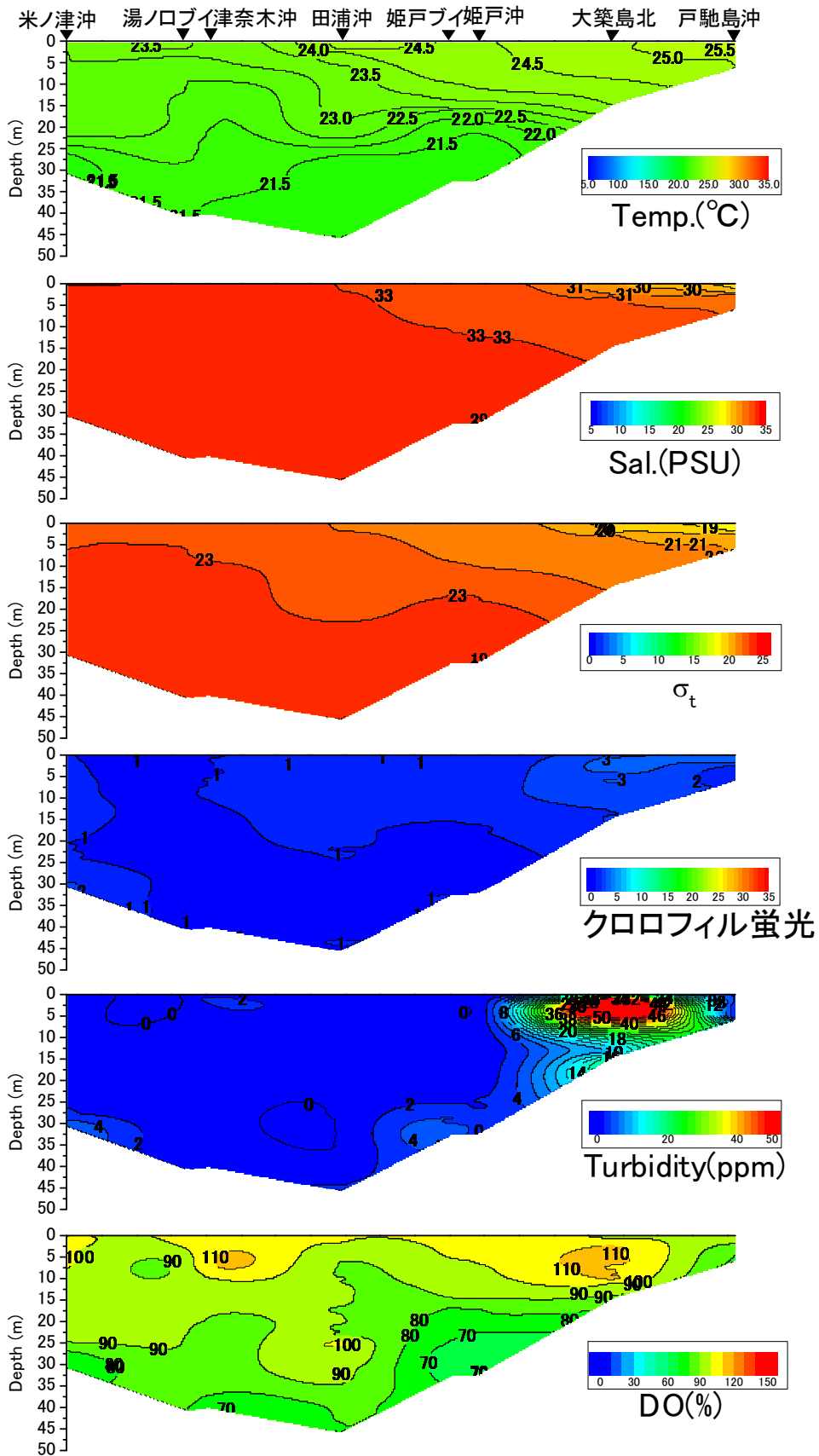
戸馳島沖から米ノ津沖の水温(°C)、塩分、密度( \sigma_t )、クロロフィル蛍光強度、濁度、溶存酸素飽和度(DO%)の鉛直面図(東町漁業協同組合の調査による) (2013年6月22日)
