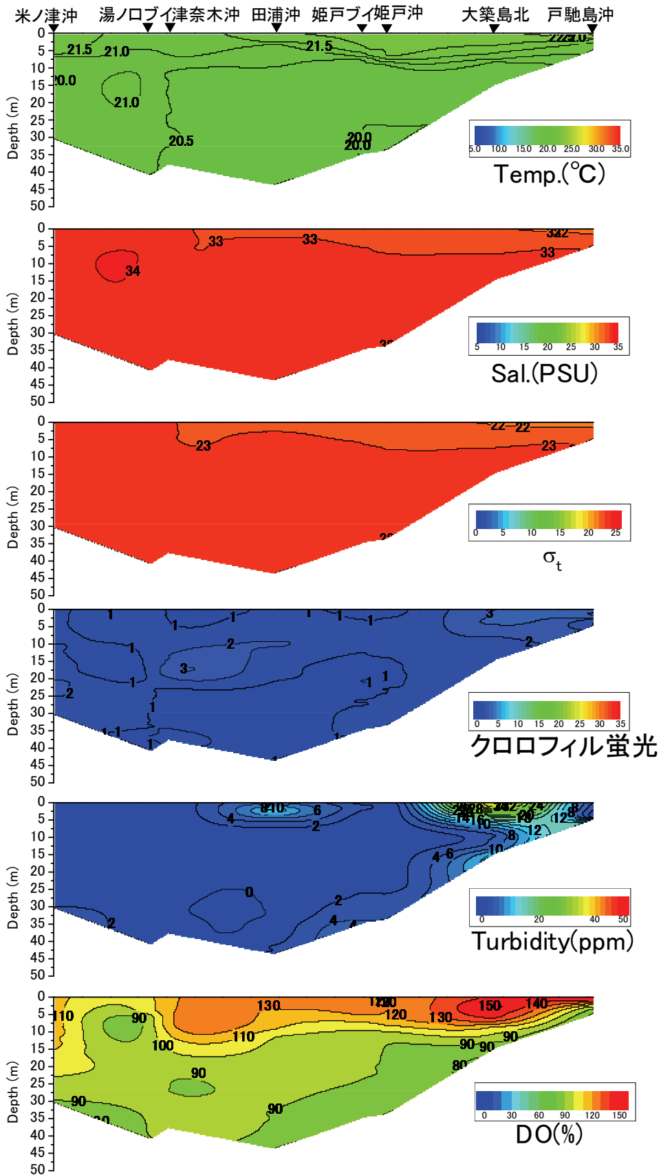
戸馳島沖から米ノ津沖の水温(°C)、塩分、密度( \sigma_t )、クロロフィル蛍光強度、濁度、溶存酸素飽和度(DO%)の鉛直面図(東町漁業協同組合の調査による) (2013年6月6日)
