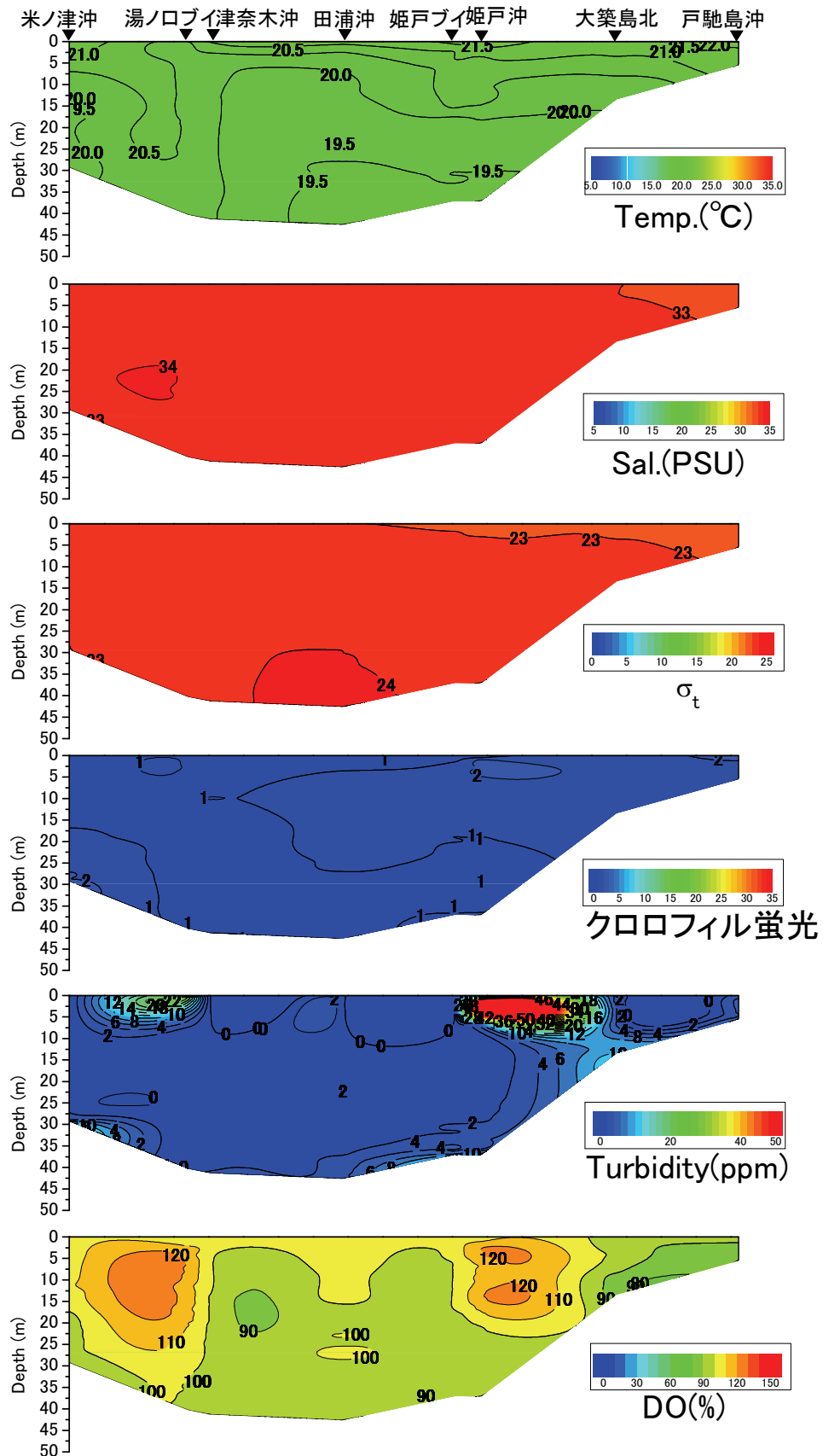
戸馳島沖から米ノ津沖の水温(°C)、塩分、密度( \sigma_t )、クロロフィル蛍光強度、濁度、溶存酸素飽和度(DO%)の鉛直面図(東町漁業協同組合の調査による) (2013年5月30日)
