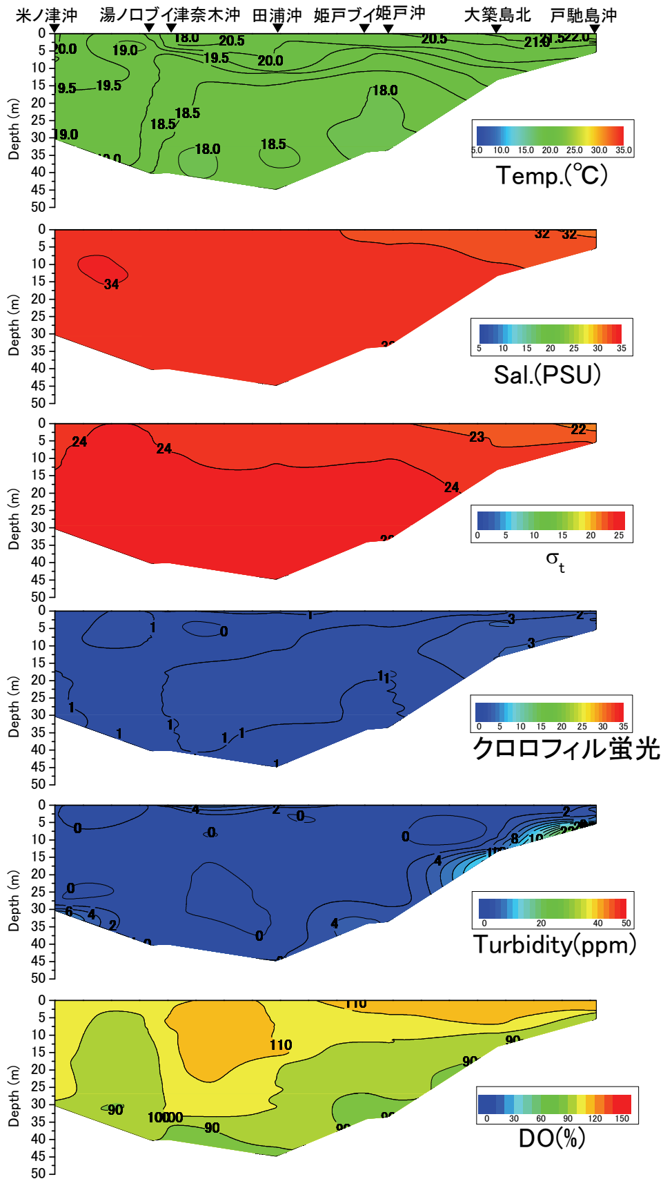
戸馳島沖から米ノ津沖の水温(°C)、塩分、密度( \sigma_t )、クロロフィル蛍光強度、濁度、溶存酸素飽和度(DO%)の鉛直面図(東町漁業協同組合の調査による) (2013年5月22日)
