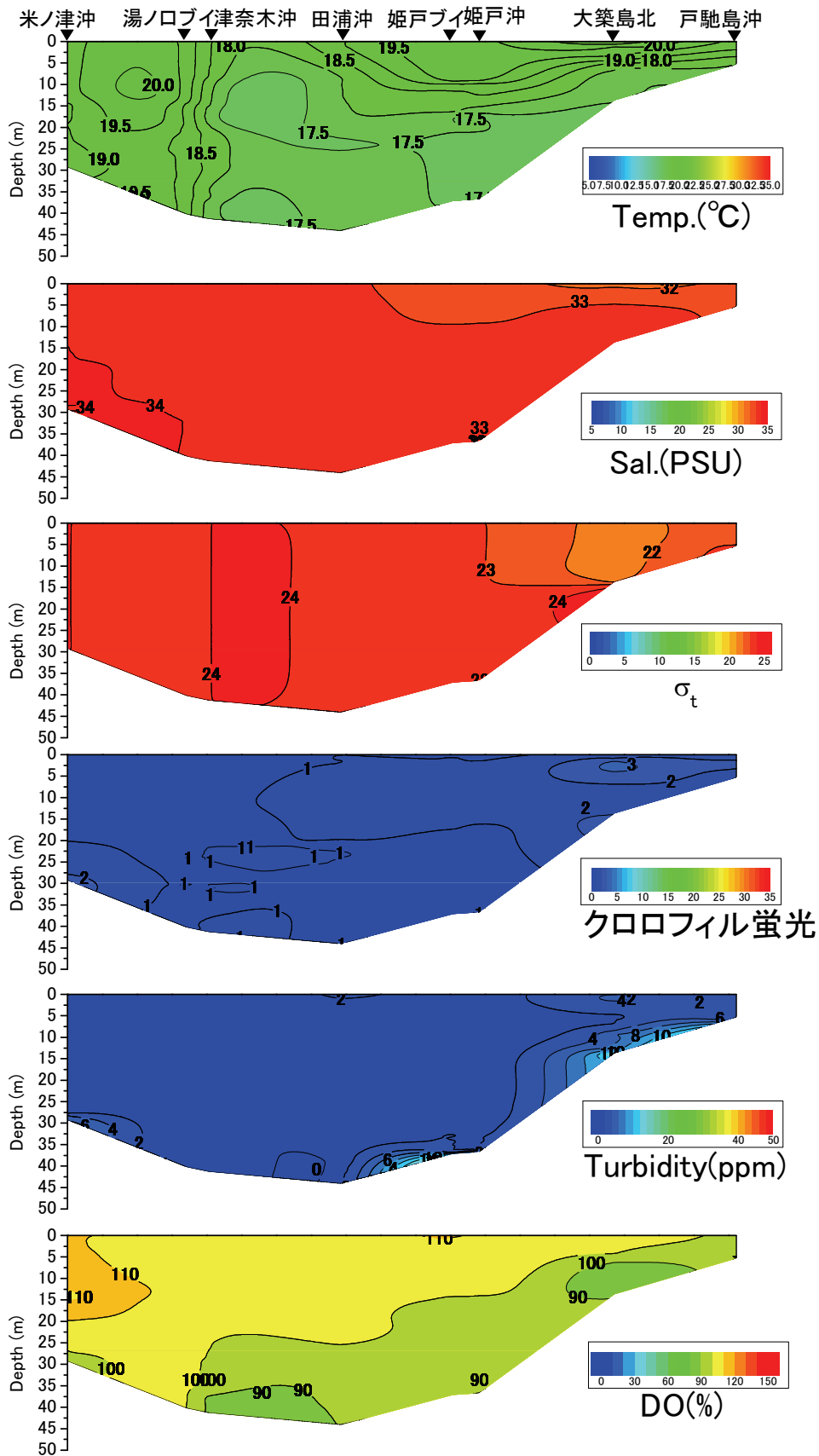
戸馳島沖から米ノ津沖の水温(°C)、塩分、密度( \sigma_t )、クロロフィル蛍光強度、濁度、溶存酸素飽和度(DO%)の鉛直面図(東町漁業協同組合の調査による) (2013年5月17日)
