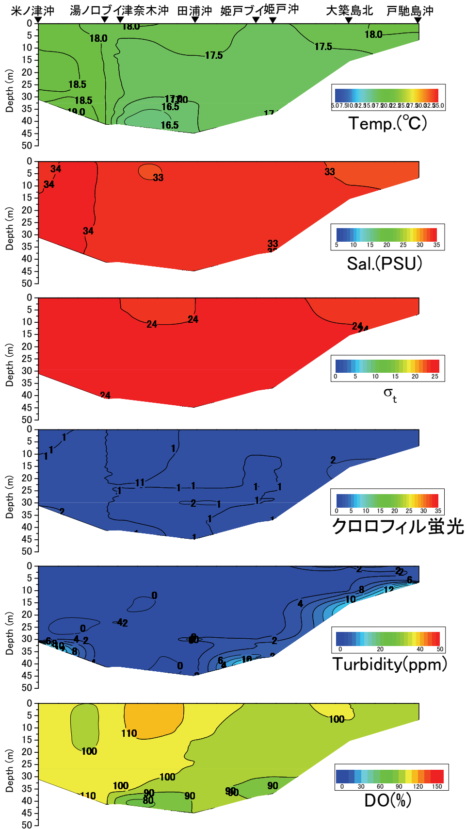
戸馳島沖から米ノ津沖の水温(°C)、塩分、密度( \sigma_t )、クロロフィル蛍光強度、濁度、溶存酸素飽和度(DO%)の鉛直面図(東町漁業協同組合の調査による) (2013年5月10日)
