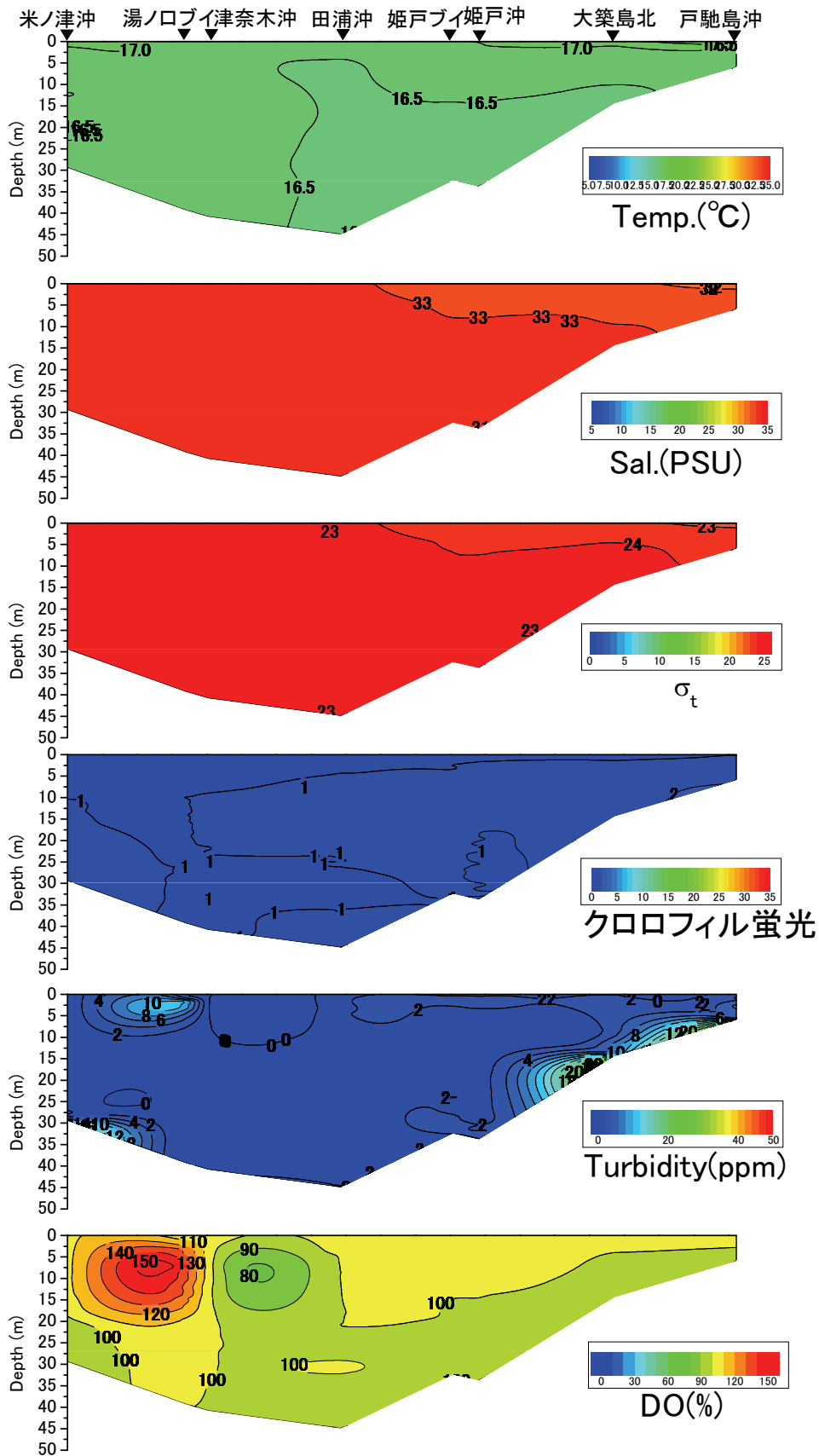
戸馳島沖から米ノ津沖の水温(°C)、塩分、密度( \sigma_t )、クロロフィル蛍光強度、濁度、溶存酸素飽和度(DO%)の鉛直面図(東町漁業協同組合の調査による) (2013年5月1日)
