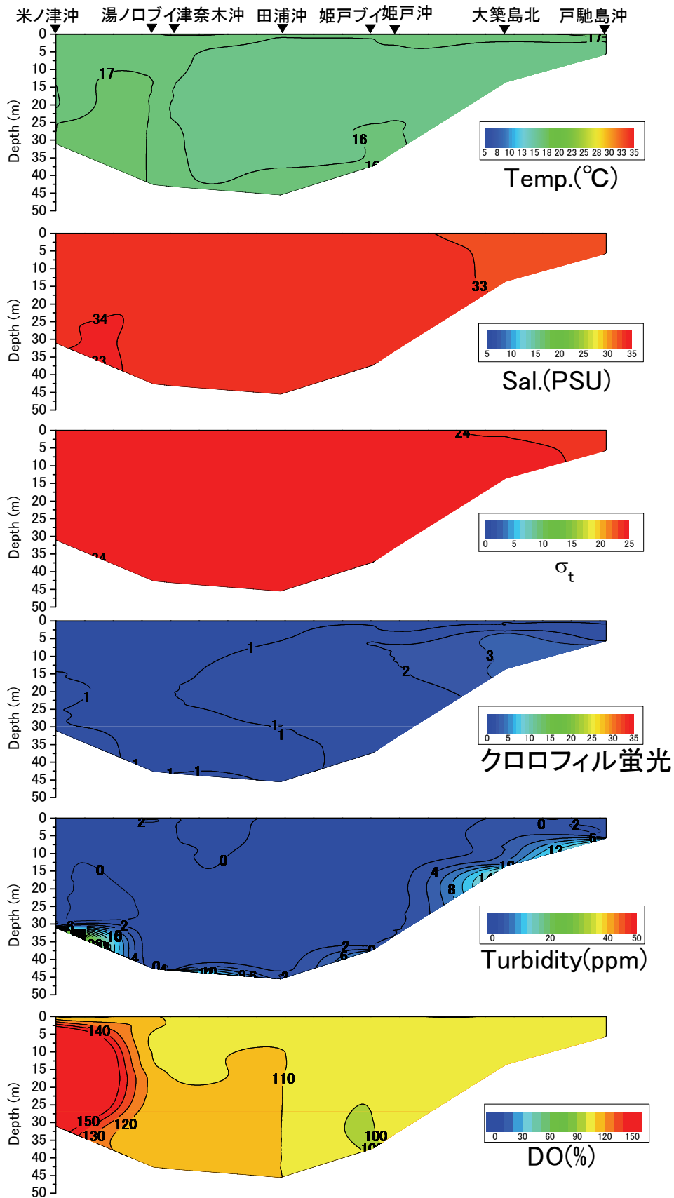
戸馳島沖から米ノ津沖の水温(°C)、塩分、密度( \sigma_t )、クロロフィル蛍光強度、濁度、溶存酸素飽和度(DO%)の鉛直面図(東町漁業協同組合の調査による) (2013年4月25日)
