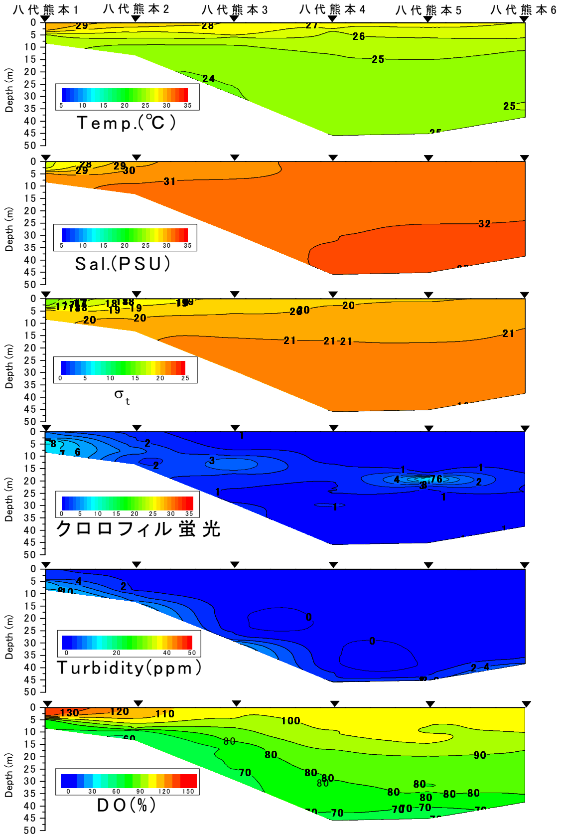
八代海東部海域の水質の断面分布 (2011年8月10日). 西海区水産研究所観測 (水産庁委託「赤潮・貧酸素水塊漁業被害防止対策事業」による)
