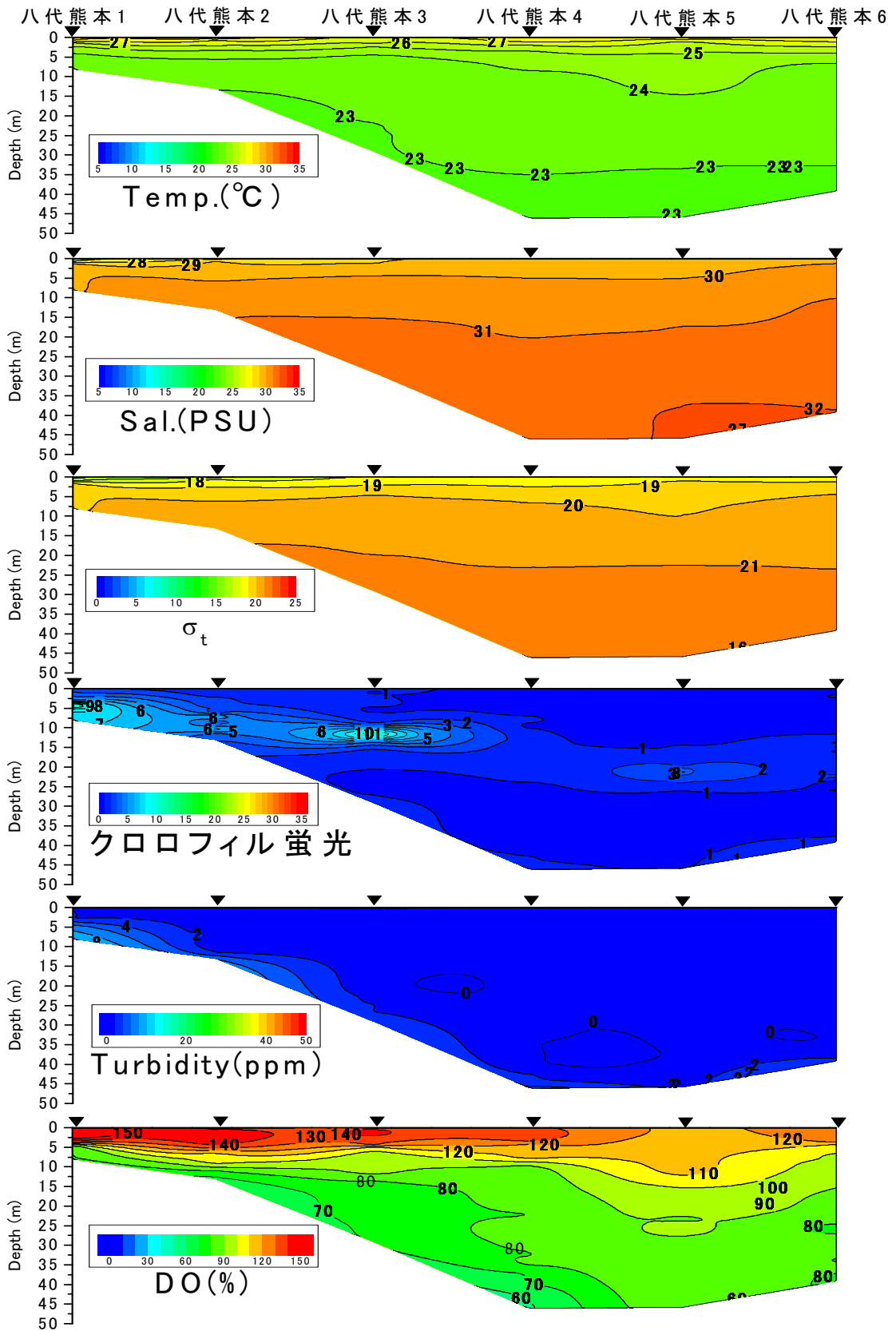
八代海東部海域の水質の断面分布 (2011年7月24日). 西海区水産研究所観測 (水産庁委託「赤潮・貧酸素水塊漁業被害防止対策事業」による)
