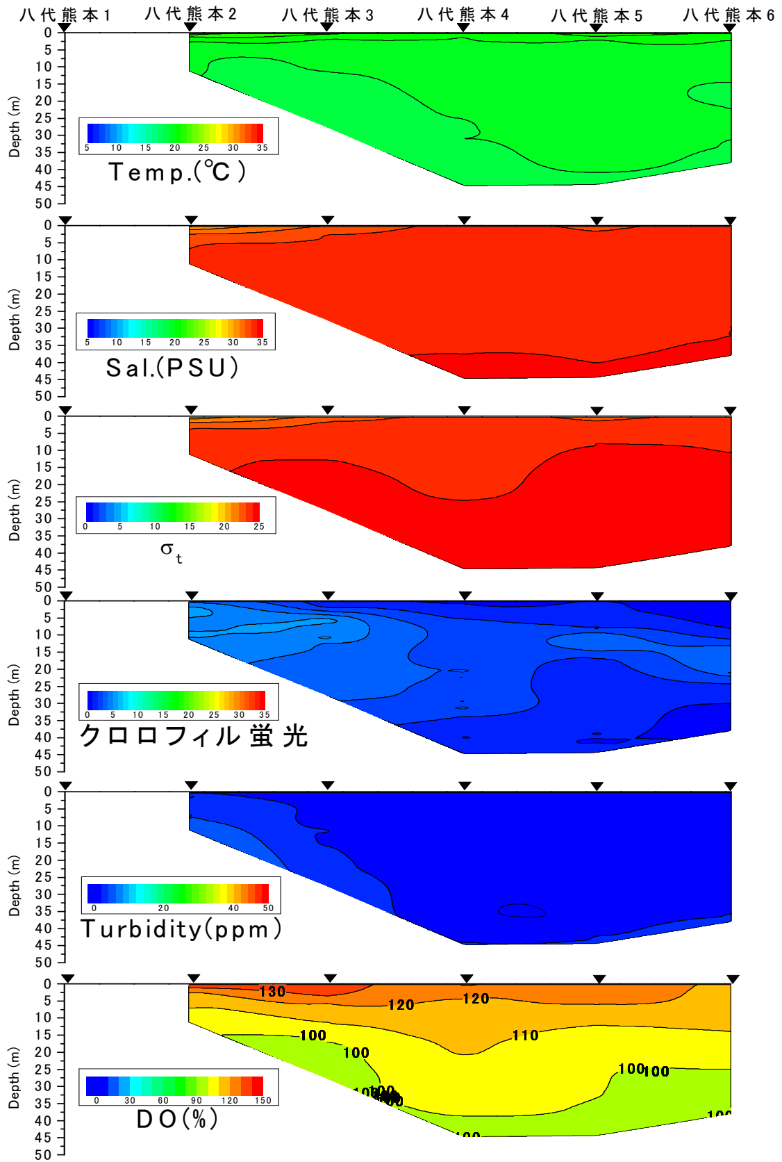
八代海東部海域の水質の断面分布 (2011年6月3日). 西海区水産研究所観測 (水産庁委託「赤潮・貧酸素水塊漁業被害防止対策事業」による)
