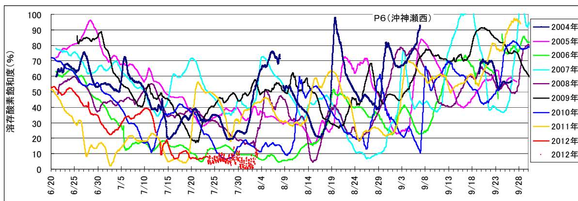
図5. 観測点P6（沖神瀬西）底層におけるの溶存酸素（25時間移動平均）の変動
