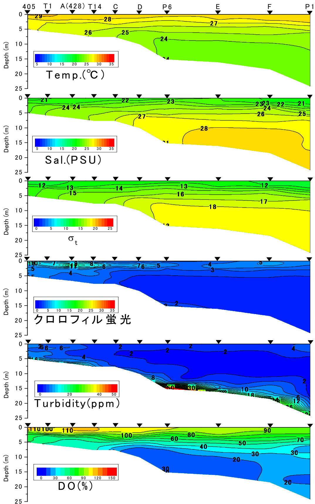
図 8. 有明海湾奥部西部海域 (図 6 の断面) の水質の鉛直分布 (2012 年 8 月 3 日)
