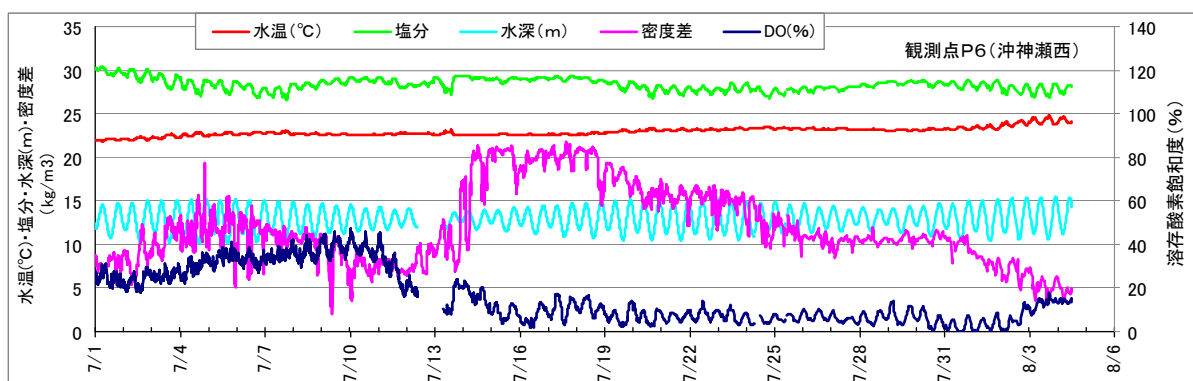
図4. 有明海奥部底層の溶存酸素等の変動（観測点P6：沖神瀬西）
