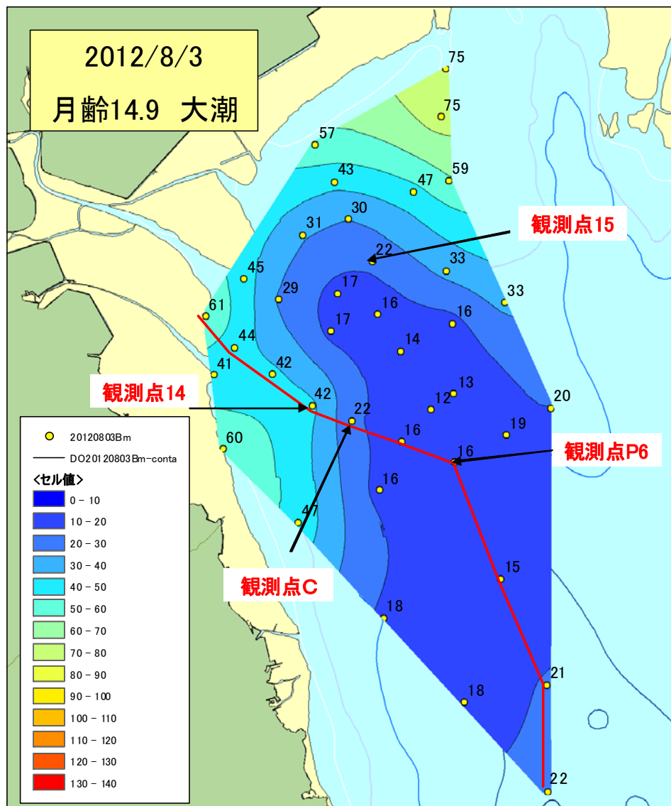
図6. 有明海湾奥部底層の溶存酸素飽和度(%)の分布(2012年8月3日)
