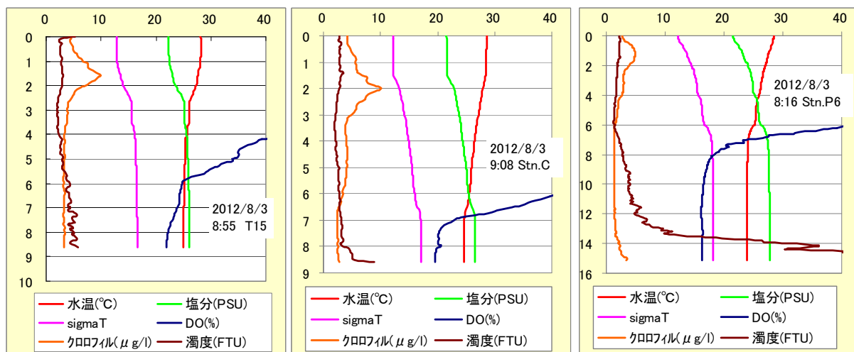
図7. 水質の鉛直分布(2012年8月3日)
