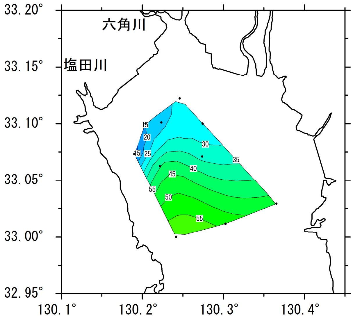
2015年8月9日 有明海奥部の海底直上0.2mの溶存酸素飽和度の水平分布 (水産庁委託及び環境省請負業務による西海区水産研究所の観測結果)
