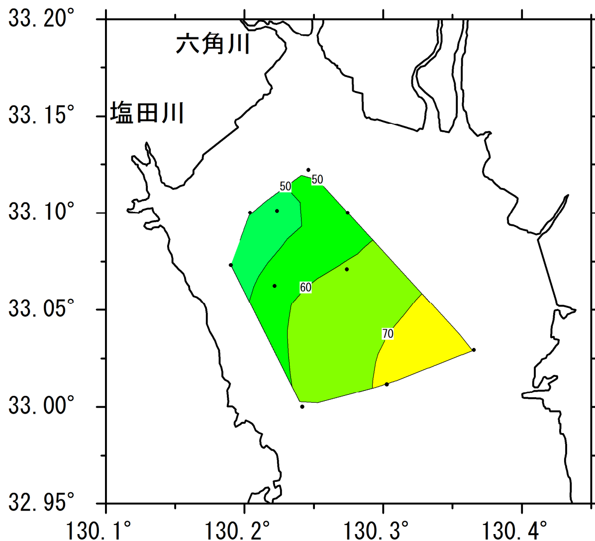
2015年6月11日 有明海奥部の海底直上0.2mの溶存酸素飽和度の水平分布 (水産庁委託及び環境省請負業務による西海区水産研究所の観測結果)
