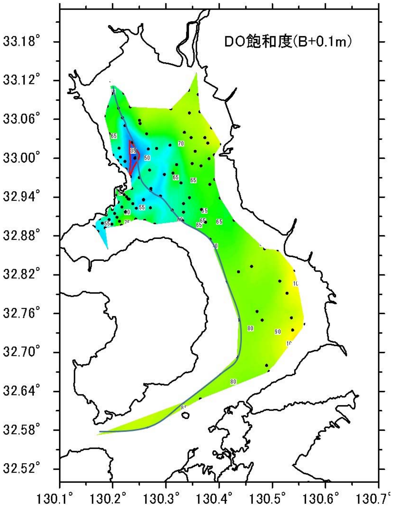
有明海一斉観測時(2014年8月5日満潮時)における底層溶存酸素飽和度の分布(17機関による)。赤線内が溶存酸素飽和度40%以下の貧酸素水塊。
