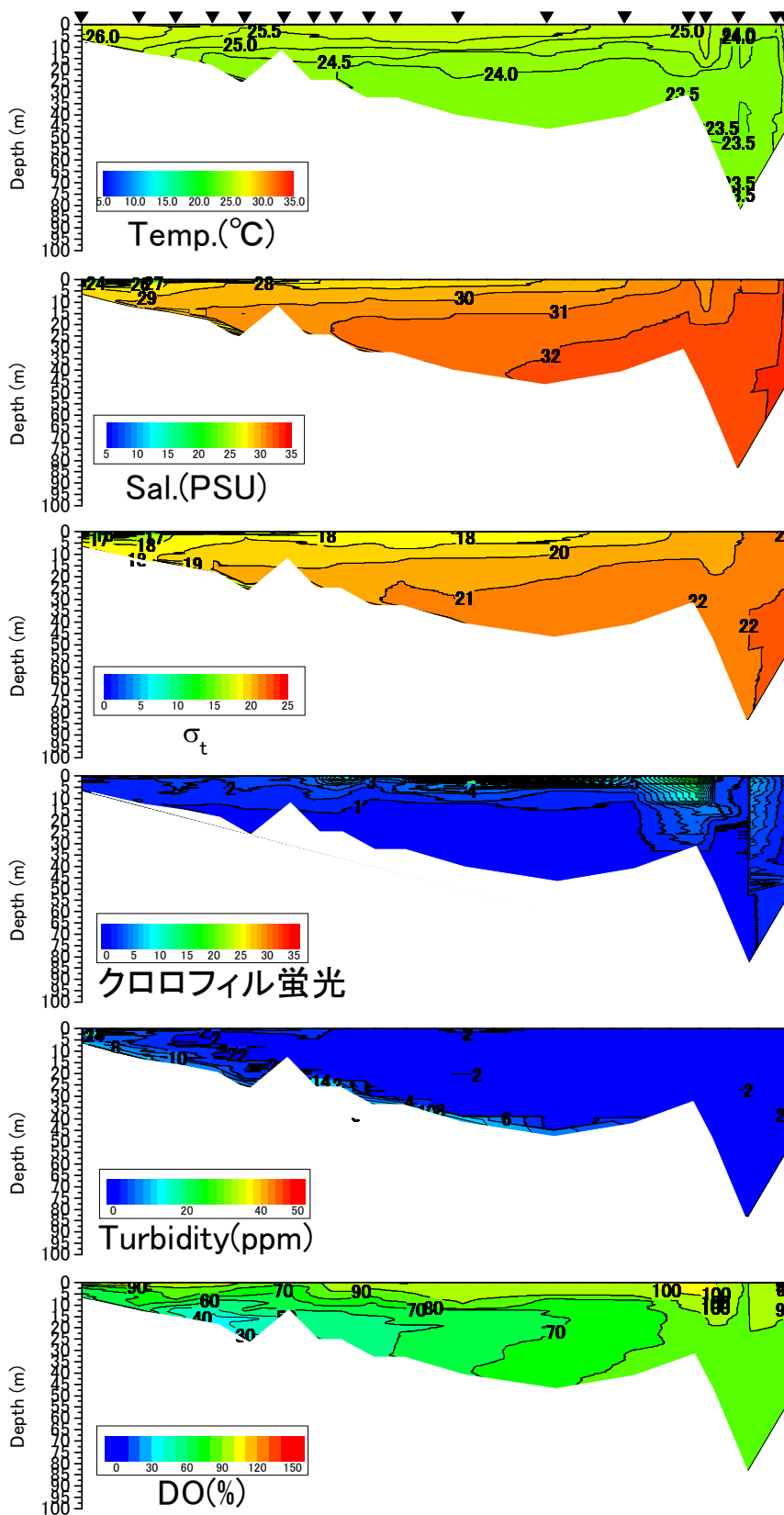
有明海一斉観測時(2014年8月5日満潮時)における水質断面図(17機関による)
