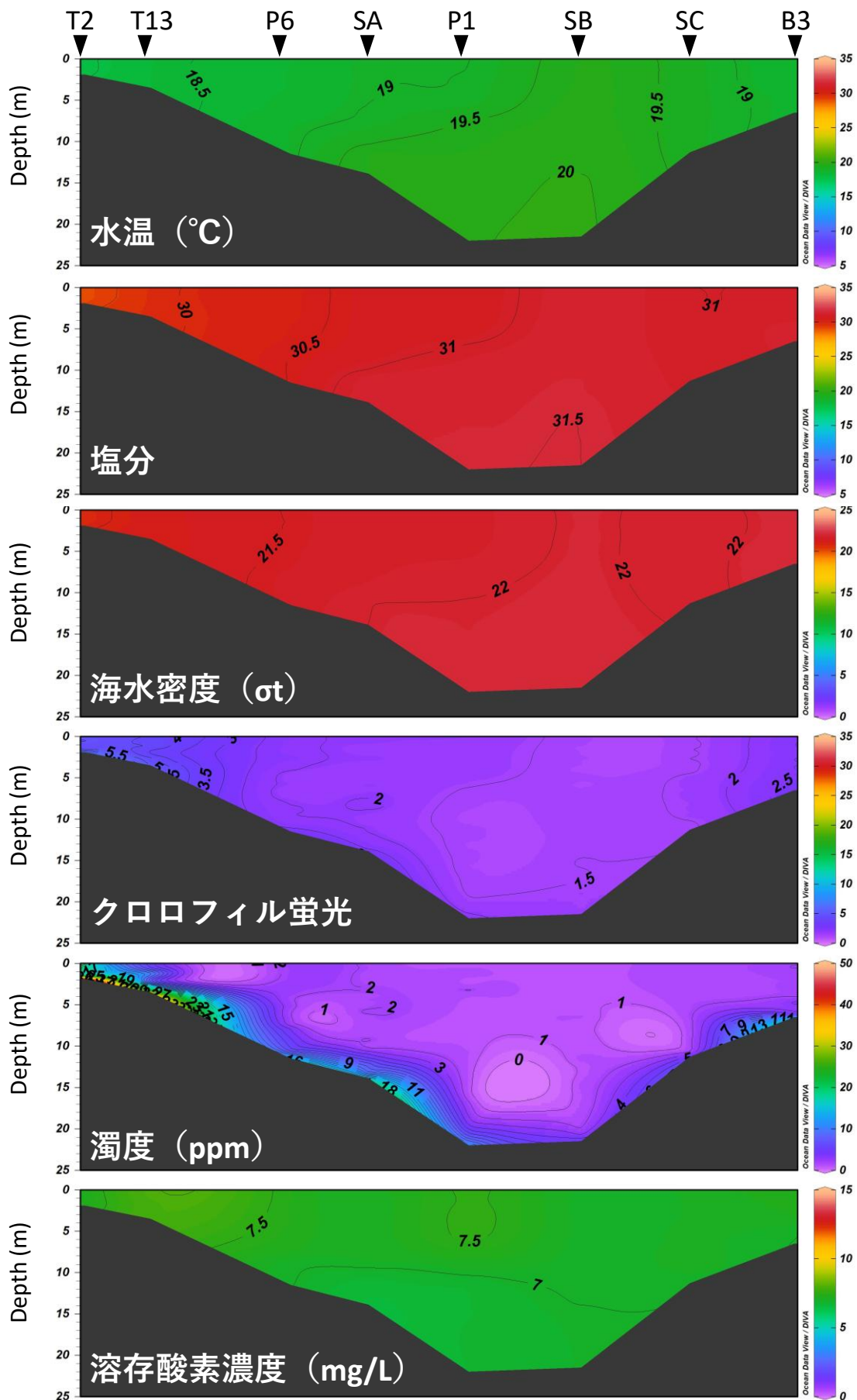
2025年11月10日における水温、塩分、密度 \sigma_t 、クロロフィル蛍光、濁度、溶存DO
