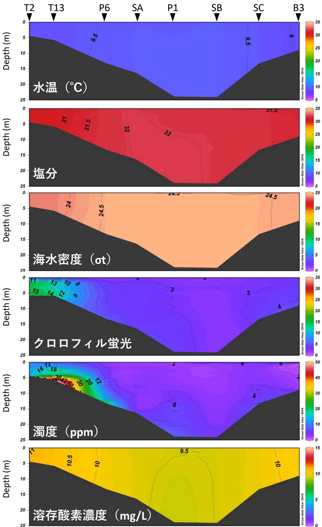
2025年2月27日における水温、塩分、密度 \sigma_t 、クロロフィル蛍光、濁度、溶存DO
