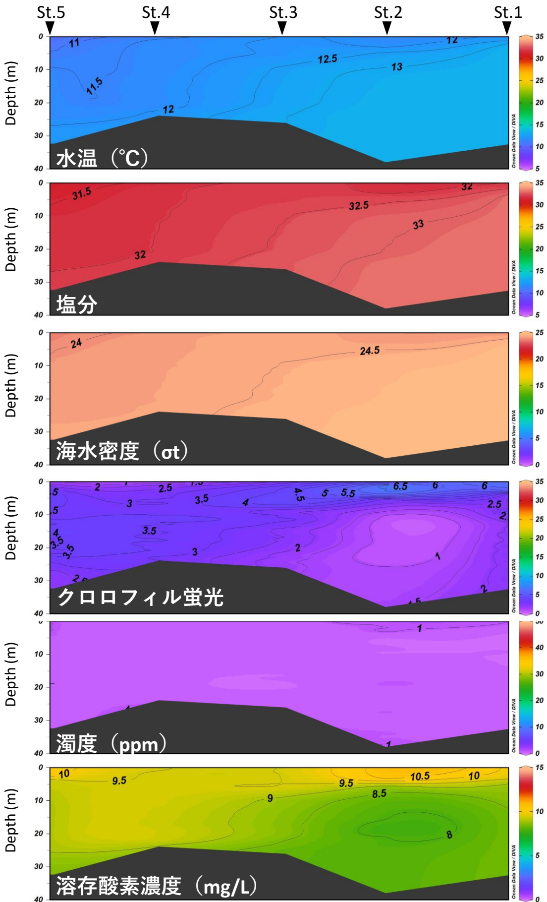
2025年1月22日における水温、塩分、密度 \sigma_t 、クロロフィル蛍光、濁度、溶存DO
