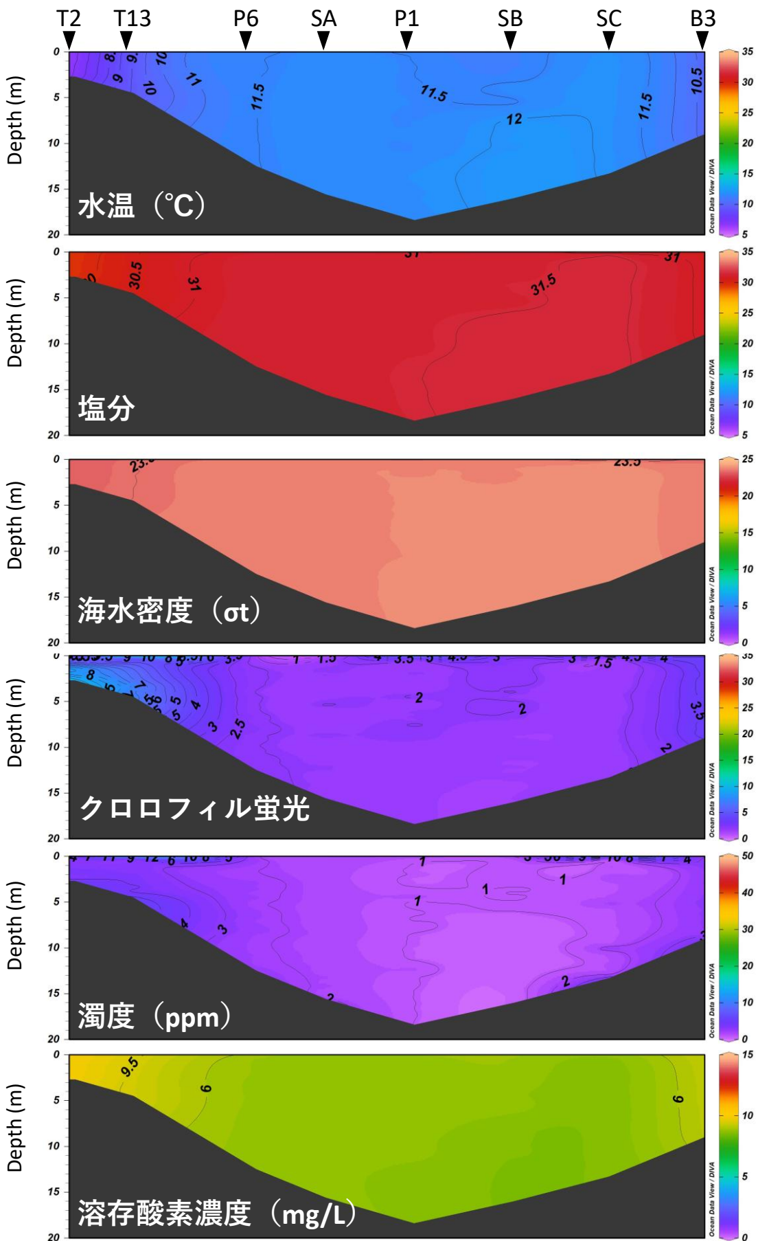
2025年1月10日における水温、塩分、密度 \sigma_t 、クロロフィル蛍光、濁度、溶存DO
