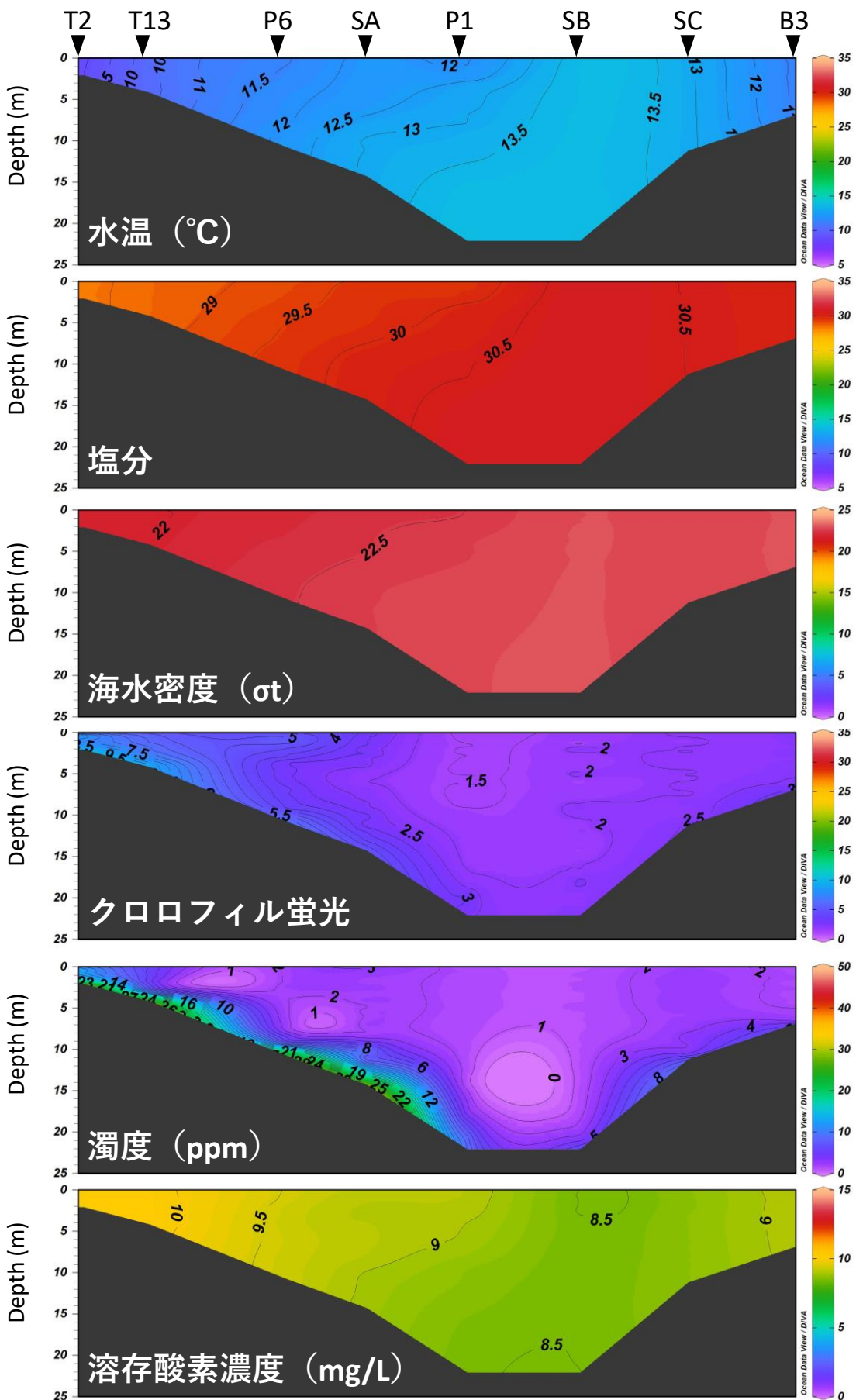
2024年12月20日における水温、塩分、密度 \sigma_t 、クロロフィル蛍光、濁度、溶存DO
