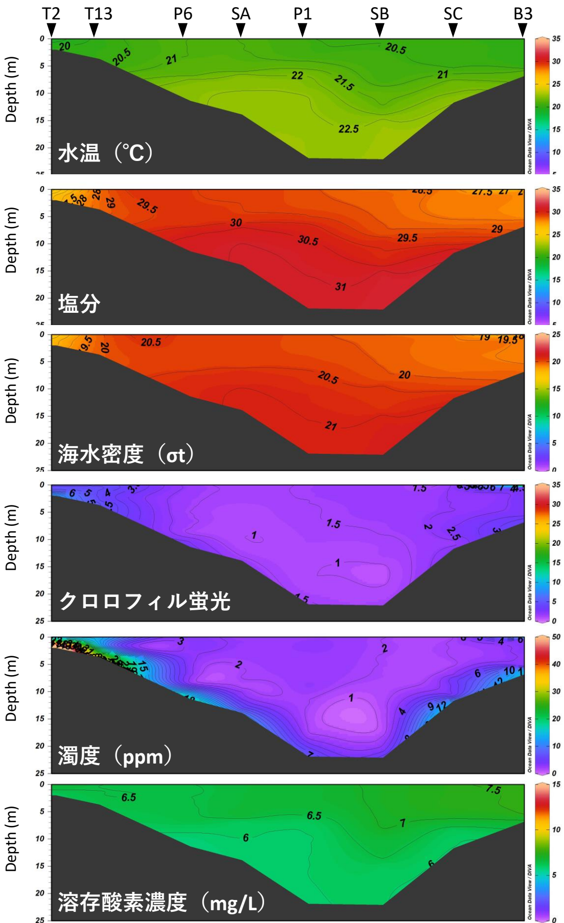
2024年11月7日における水温、塩分、密度 \sigma_t 、クロロフィル蛍光、濁度、溶存DO
