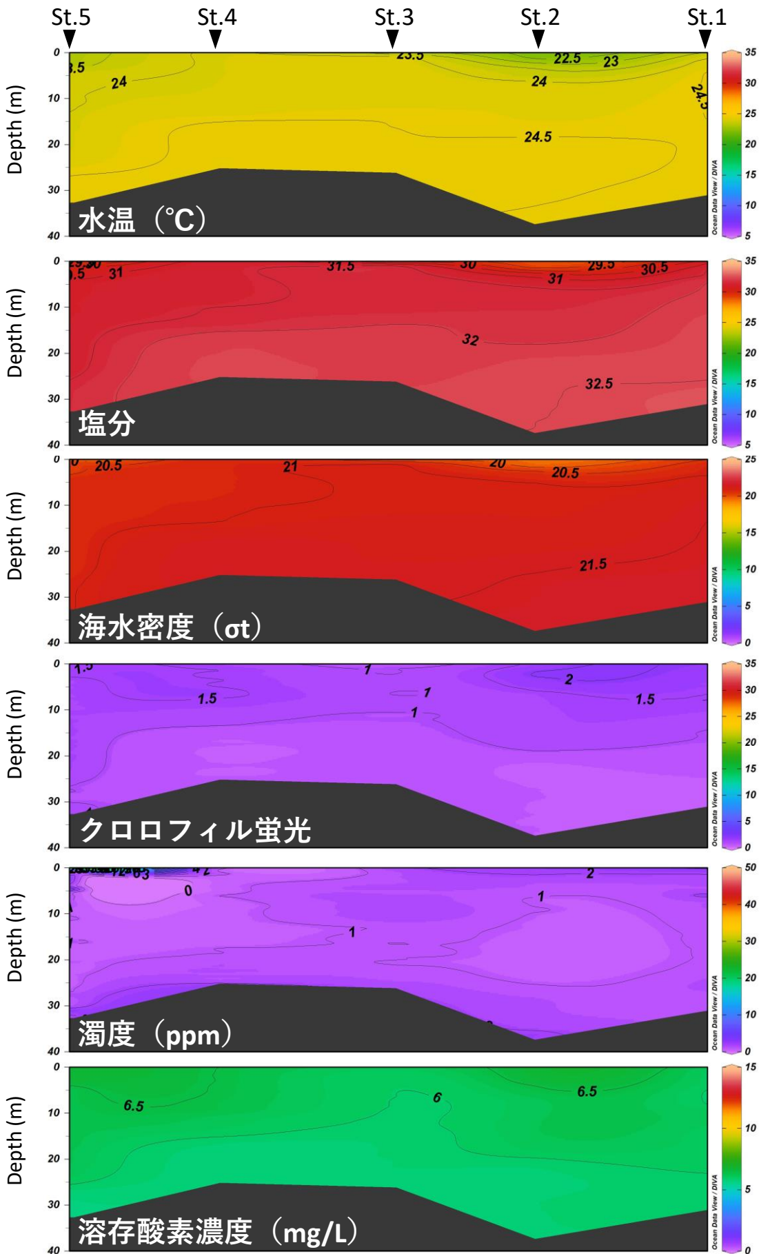
2024年10月24日における水温、塩分、密度 \sigma_t 、クロロフィル蛍光、濁度、溶存DO
