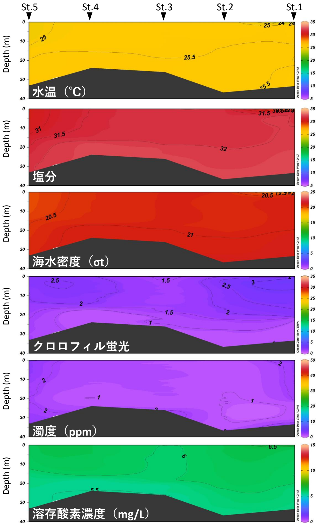
2024年10月11日における水温、塩分、密度 \sigma_t 、クロロフィル蛍光、濁度、溶存DO
