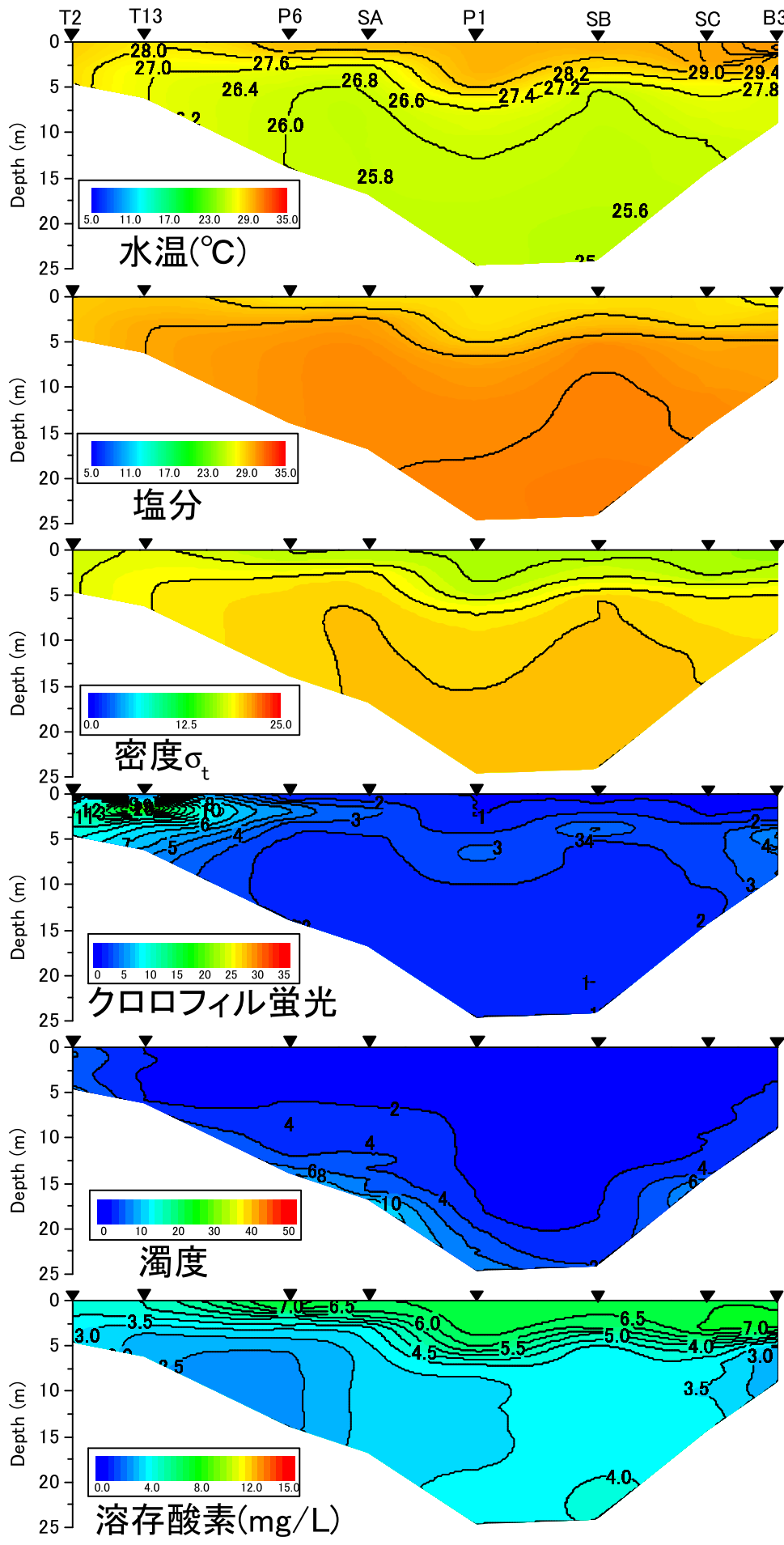
2024年8月19日における水温、塩分、密度 \sigma_t 、クロロフィル蛍光、濁度、溶存酸素
