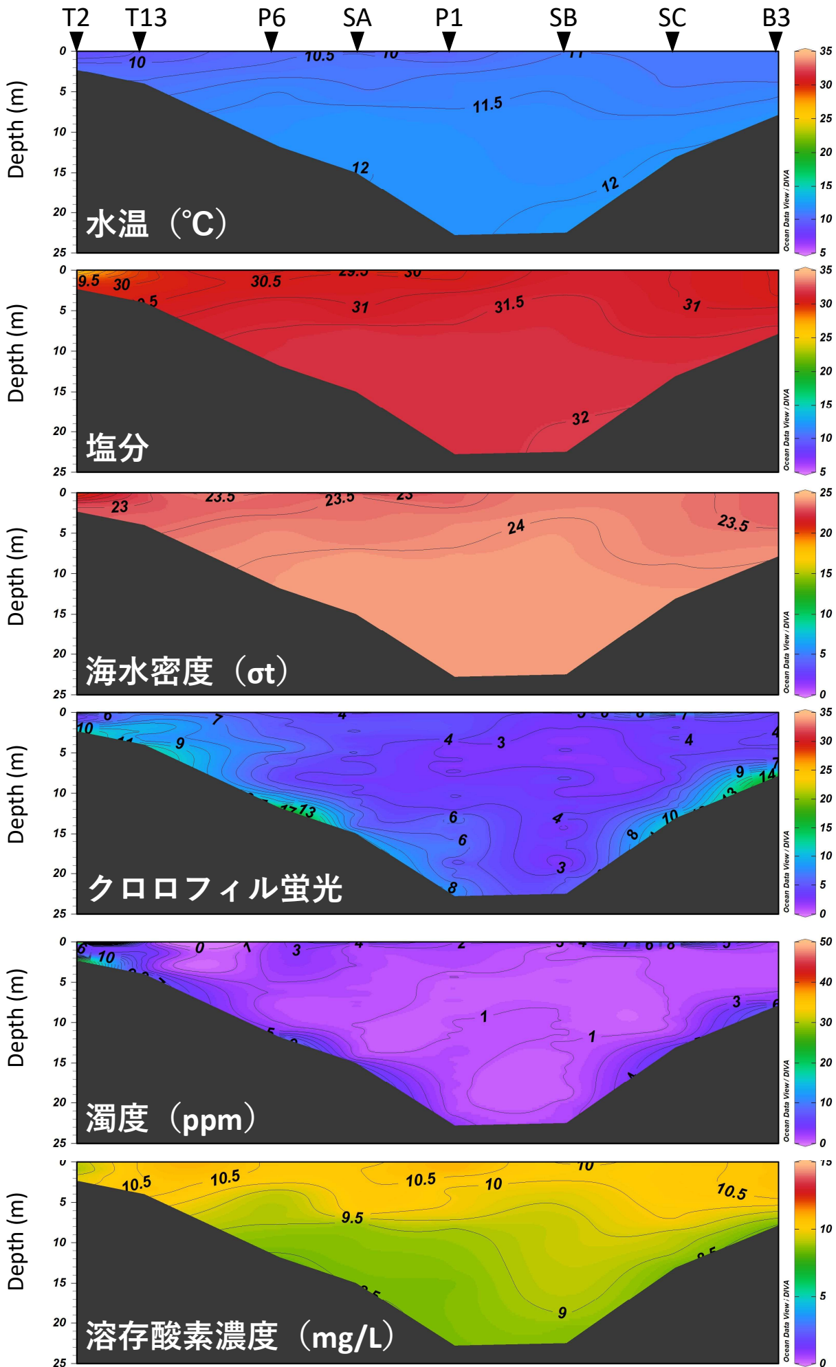
2024年3月4日における水温、塩分、密度 \sigma_t 、クロロフィル蛍光、濁度、溶存DO
