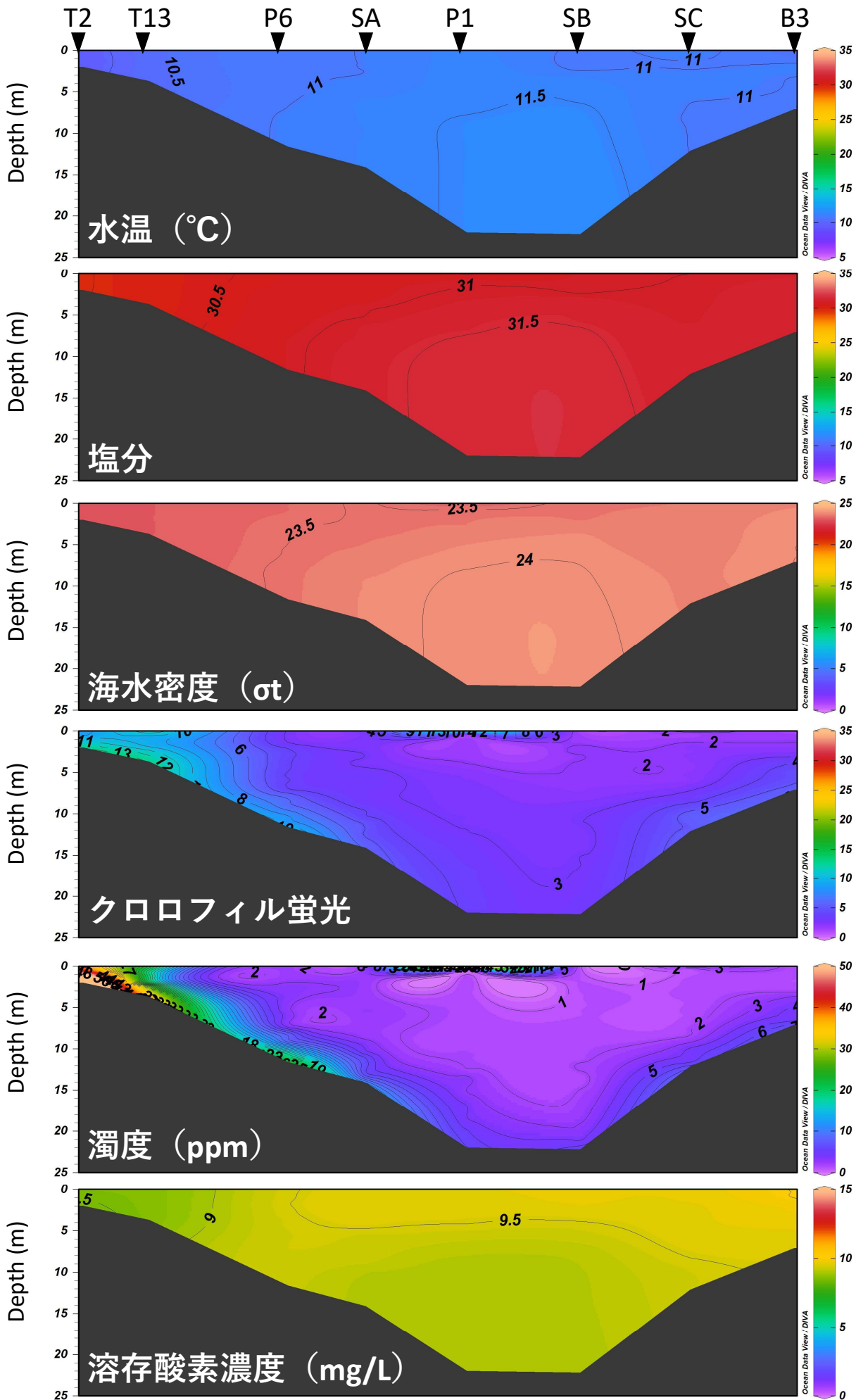
2024年1月18日における水温、塩分、密度 \sigma_t 、クロロフィル蛍光、濁度、溶存DO
