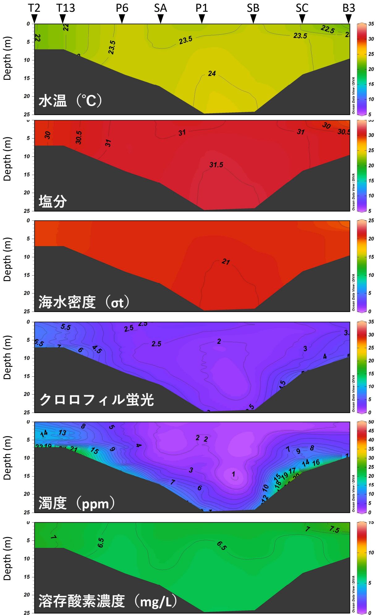
2023年10月15日における水温、塩分、密度 \sigma_t 、クロロフィル蛍光、濁度、溶存DO
