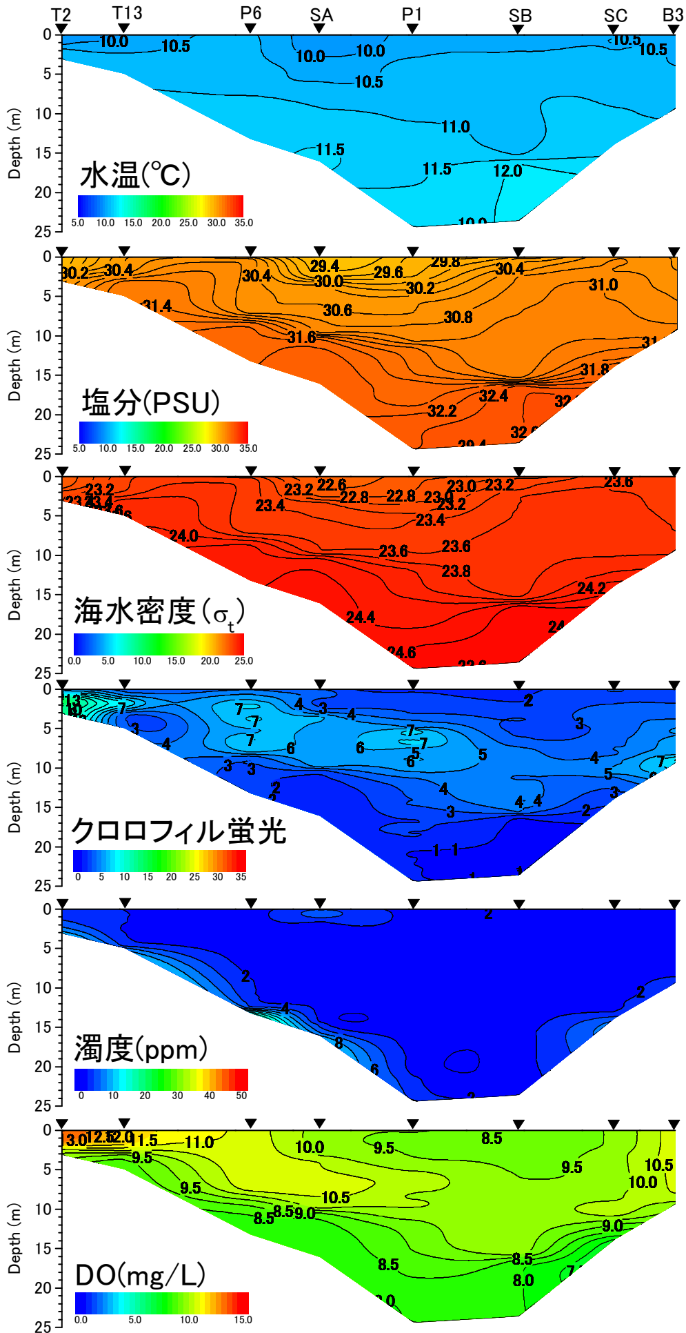
2023年3月3日における水温、塩分、密度 \sigma_t 、クロロフィル蛍光値、濁度、DO濃度
