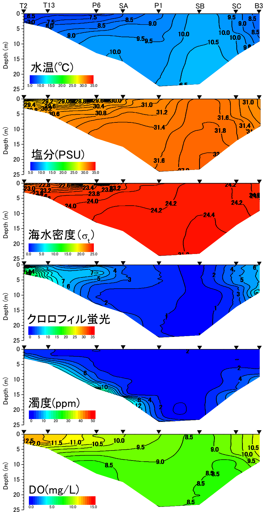
2023年2月1日における水温、塩分、密度 \sigma_t 、クロロフィル蛍光値、濁度、DO濃度
