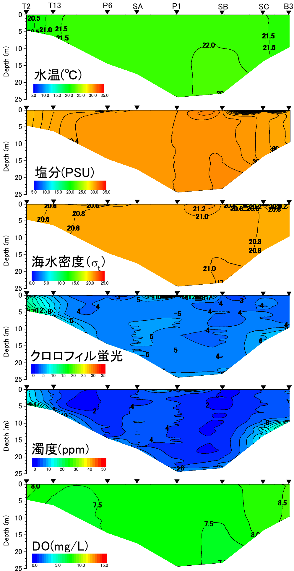
2022年10月25日における水温、塩分、密度 \sigma_t 、クロロフィル蛍光値、濁度、DO濃度
