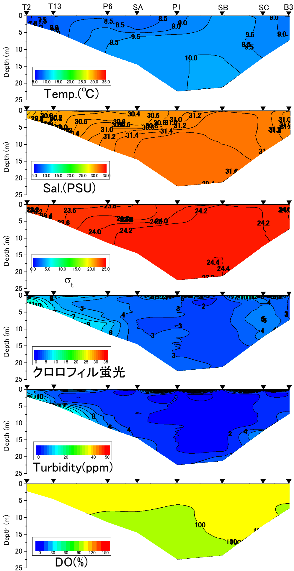
2022年2月8日における水温、塩分、密度 \sigma_t 、クロロフィル蛍光値、濁度、DO飽和度
