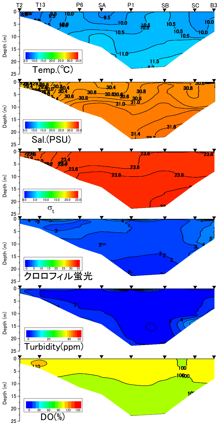
2022年1月11日における水温、塩分、密度 \sigma_t 、クロロフィル蛍光値、濁度、DO飽和度
