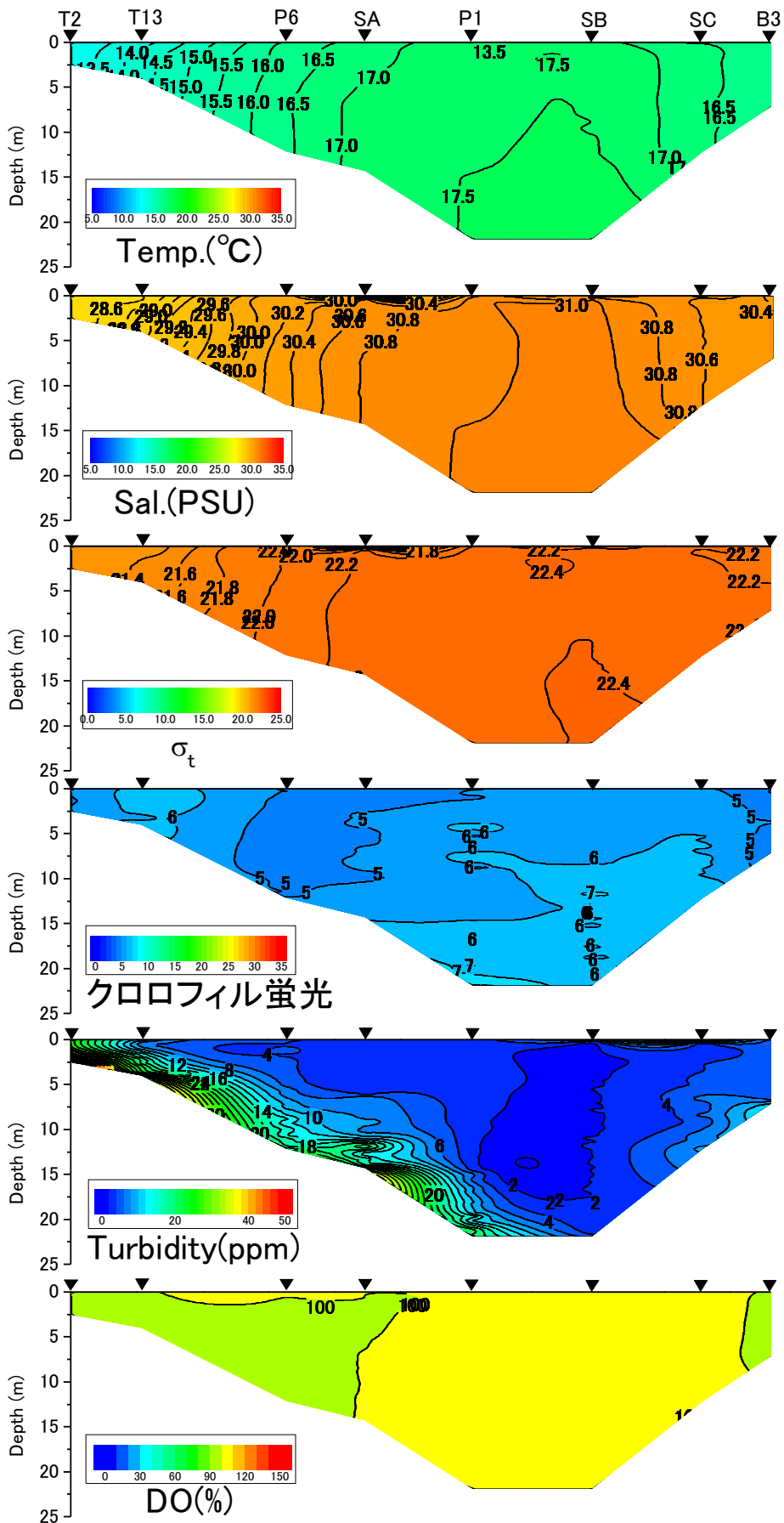
2021年11月24日における水温、塩分、密度 \sigma_t 、クロロフィル蛍光値、濁度、DO飽和度
