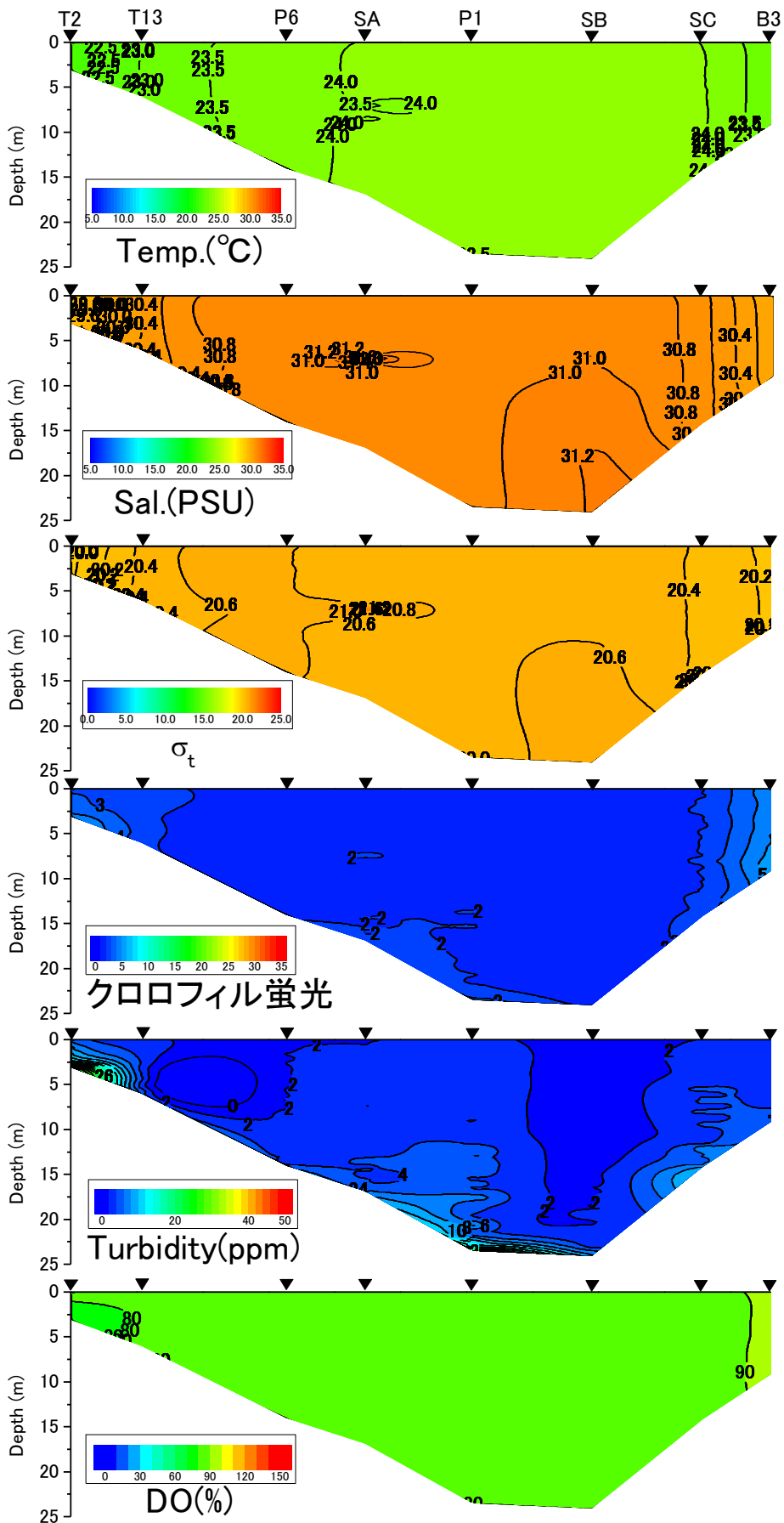
2021年10月19日における水温、塩分、密度 \sigma_t 、クロロフィル蛍光値、濁度、DO飽和度
