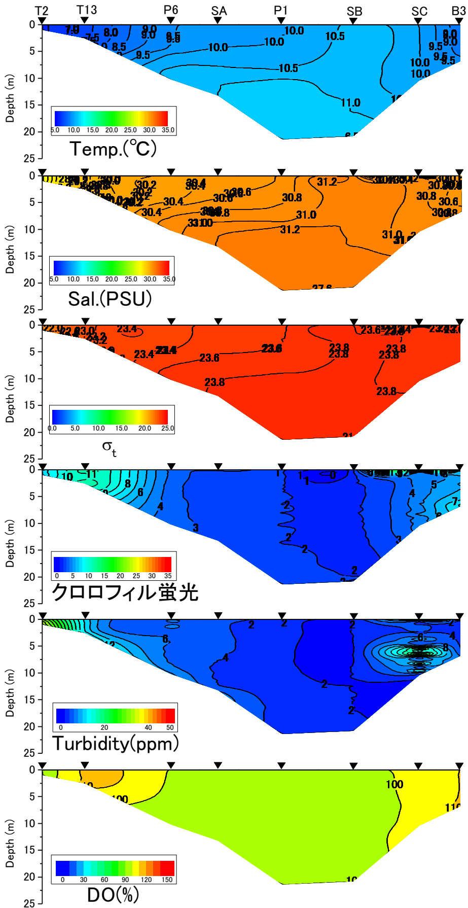
2021年1月6日における水温、塩分、密度 \sigma_t 、クロロフィル蛍光値、濁度、DO飽和度
