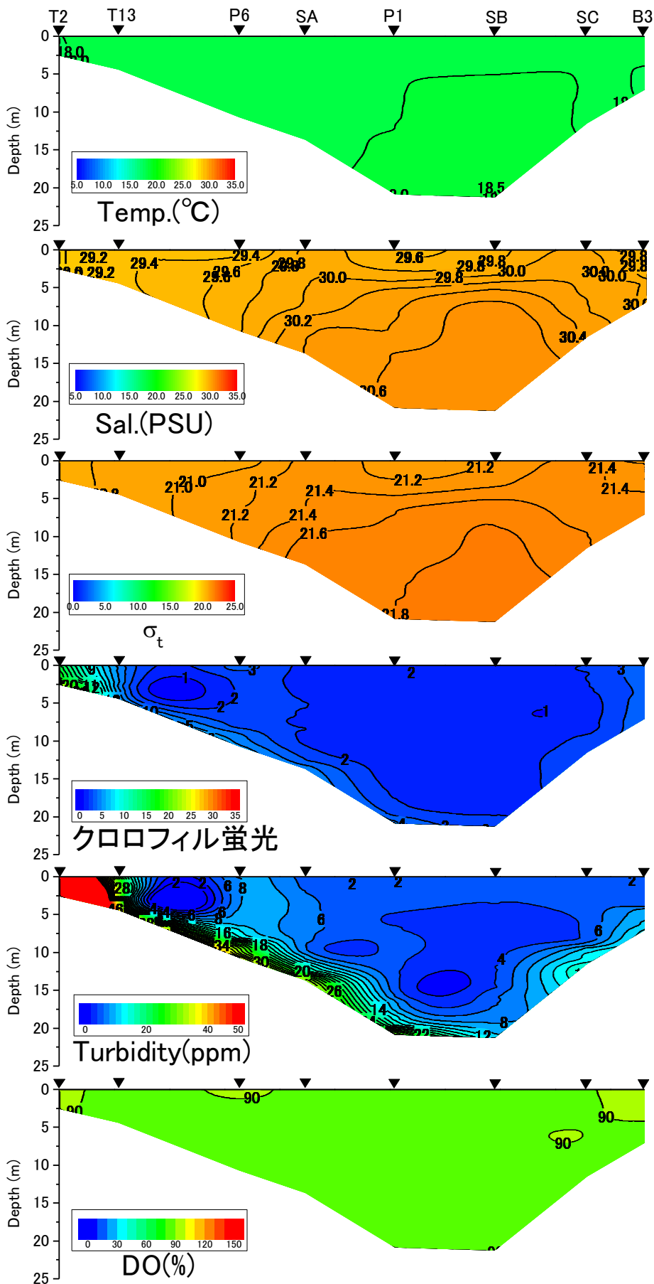
2020年11月19日における水温、塩分、密度 \sigma_t 、クロロフィル蛍光値、濁度、DO飽和度
