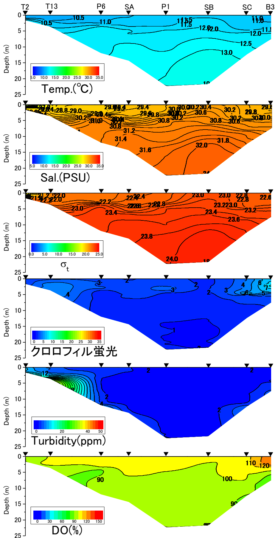
2020年2月3日における水温、塩分、密度 \sigma_t 、クロロフィル蛍光値、濁度、DO飽和度
