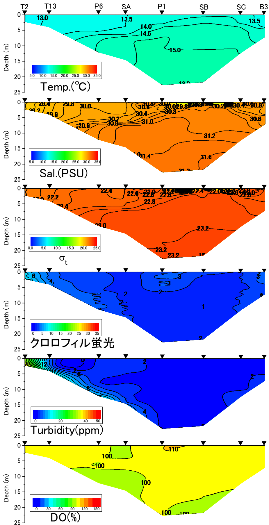
2019年12月19日における水温、塩分、密度 \sigma_t 、クロロフィル蛍光値、濁度、DO飽和度
